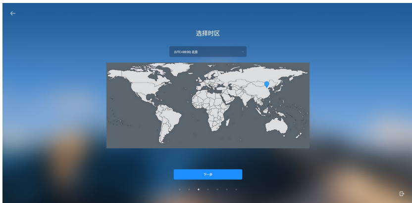
图 4 选择时区
