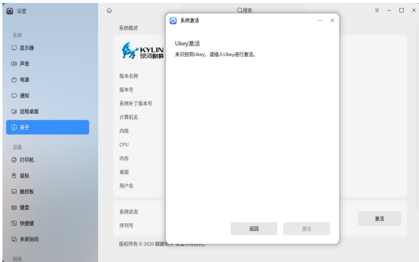
图 33 Ukey 激活
