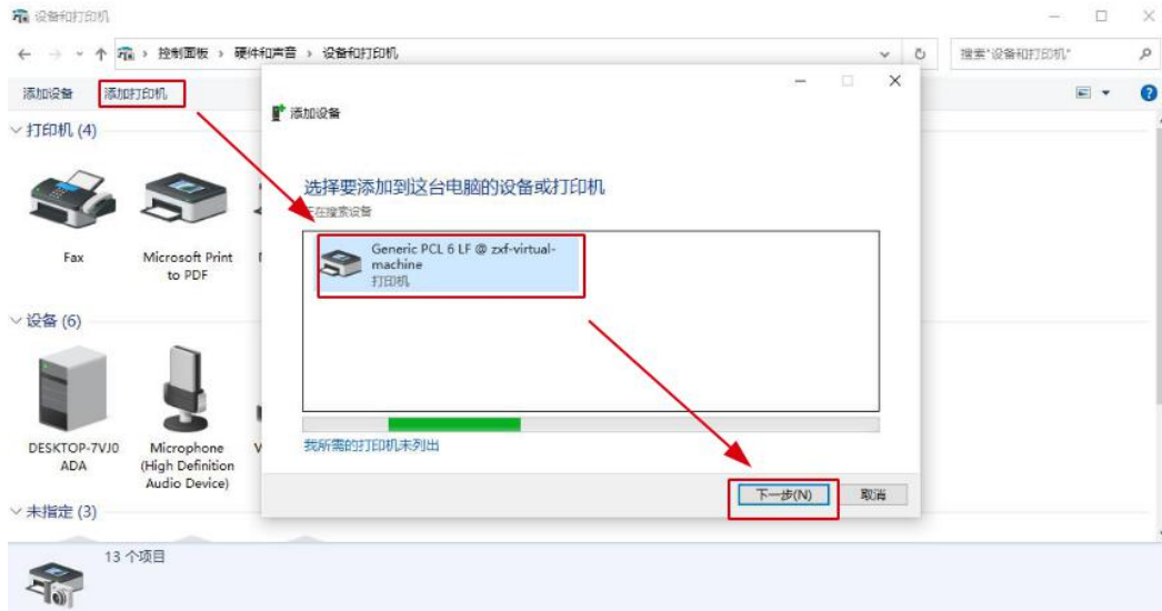
图 2.56 添加打印机
