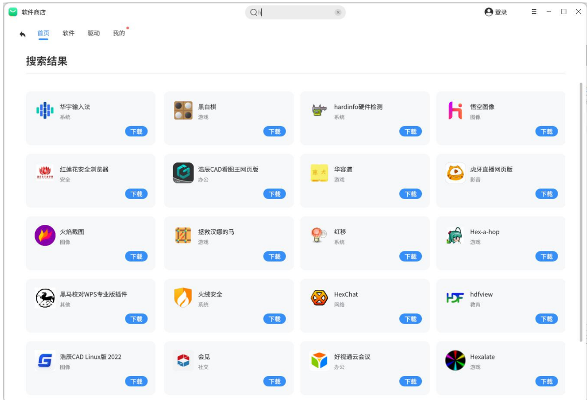
图 3.27 搜索结果
