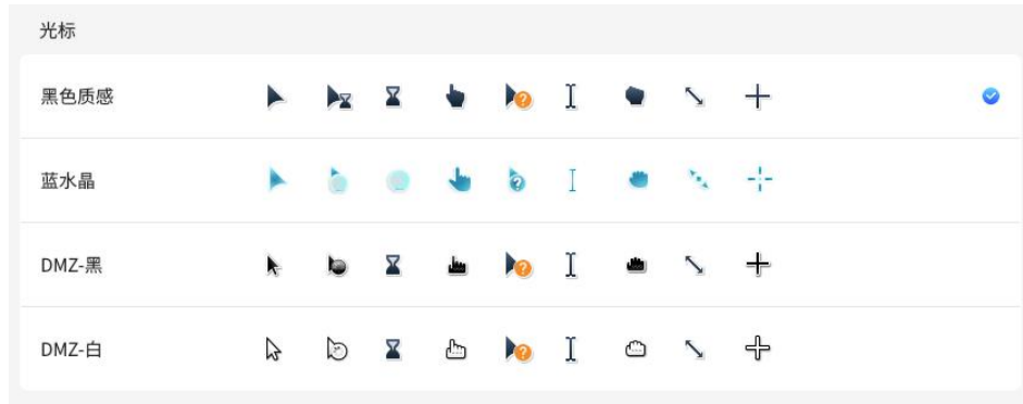
图 2.10 光标主题
