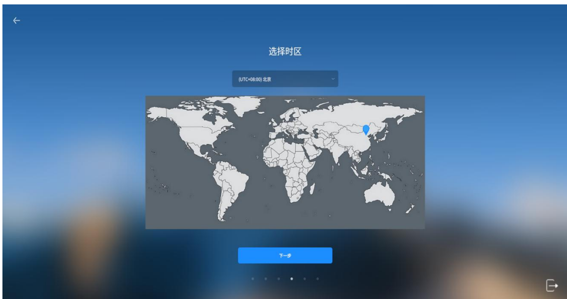
图 5 选择时区
