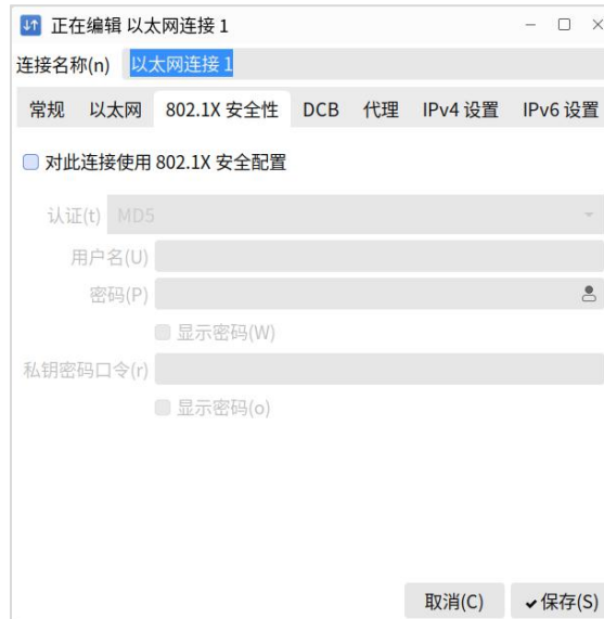
图 2.93 802.1X 安全性
