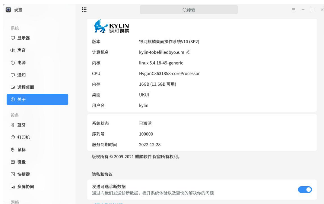
图 1.3 系统概述
