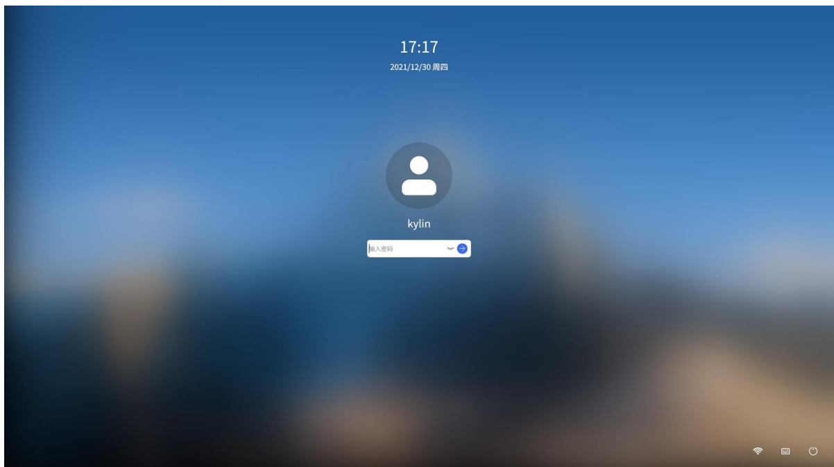
图 1.1 登录界面
