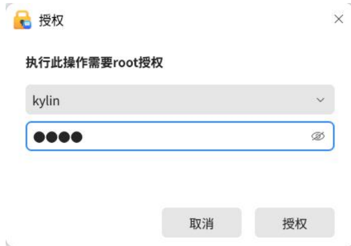
图 3.64 执行授权
