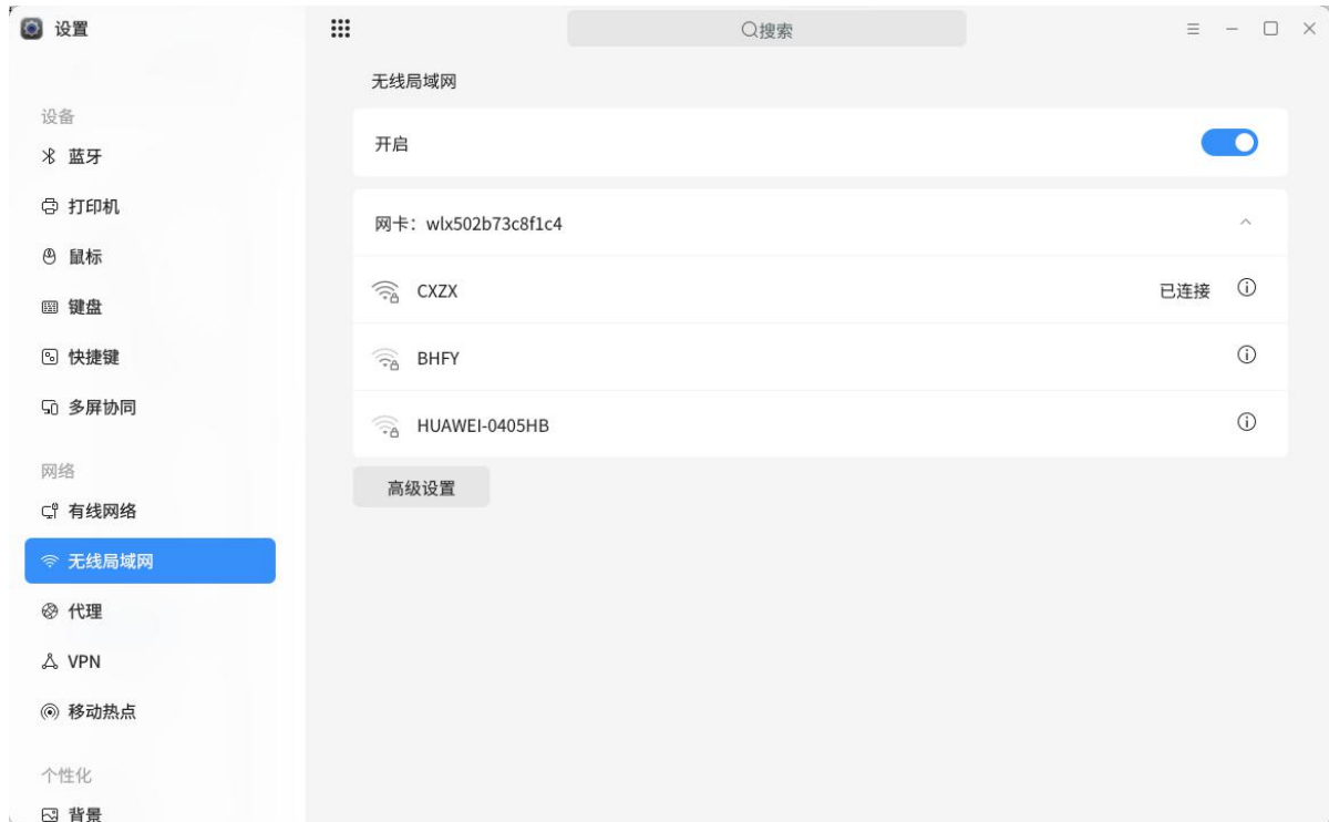
图 2.116 无线局域网
