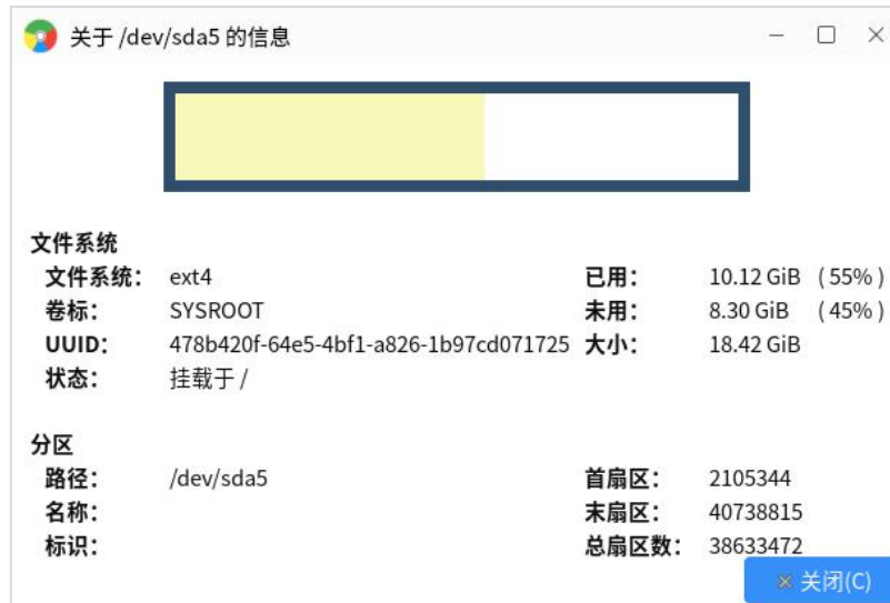
图 5.55 信息
