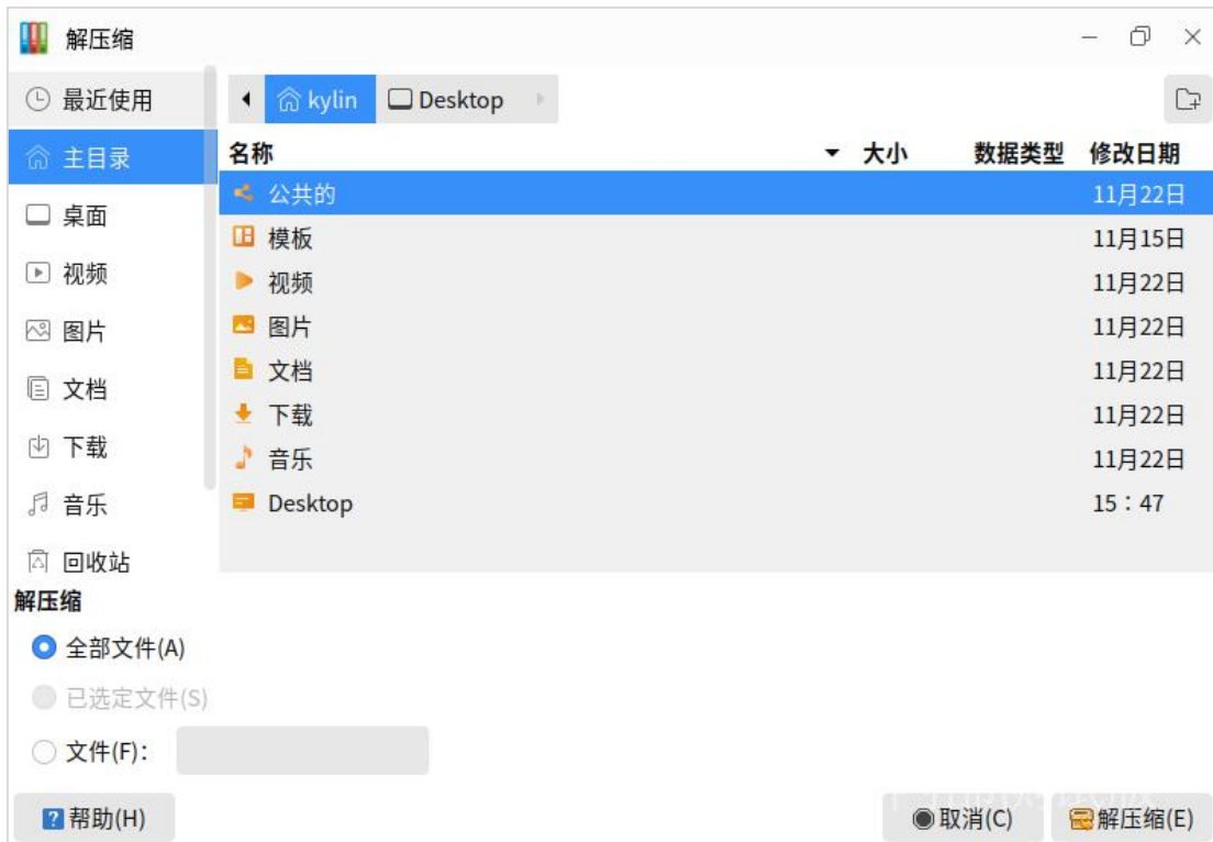
图 3.182 选择路径
