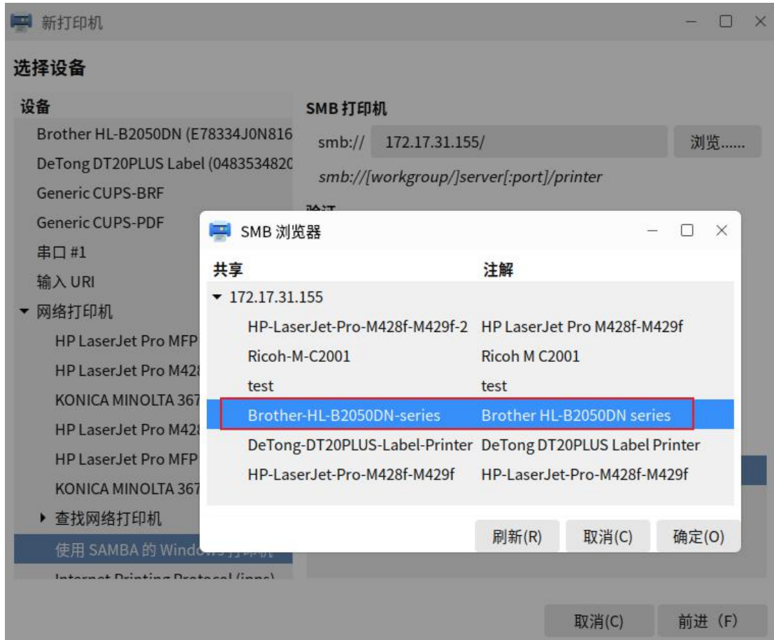
图 2.53 选择设备
