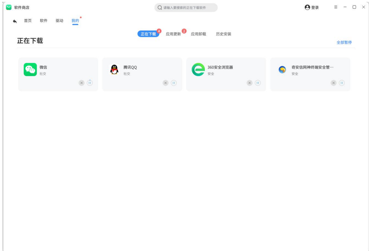
图 3.19 正在下载
