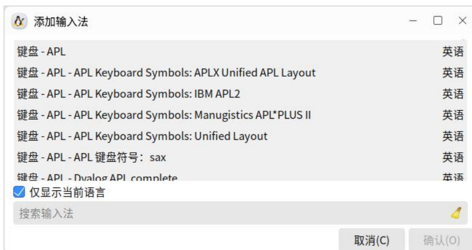
图 3.3 添加输入法
