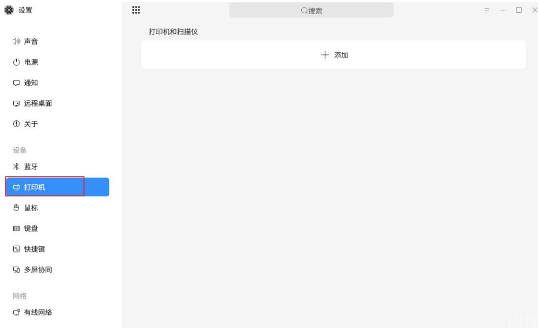
图 2.22 打印机
