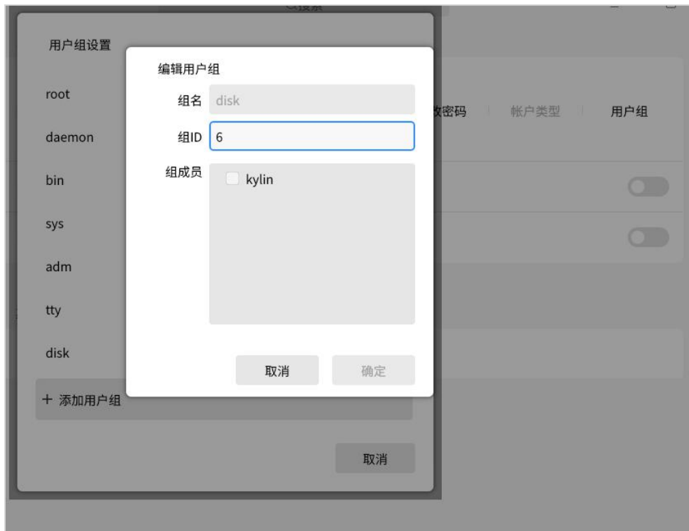
图 2.131 用户组操作
