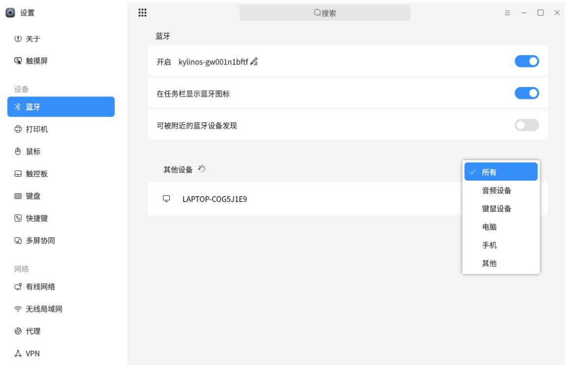
图 2.13 筛选设备
