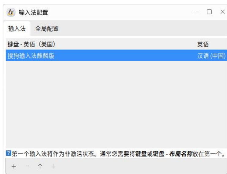
图 2.69 输入法配置
