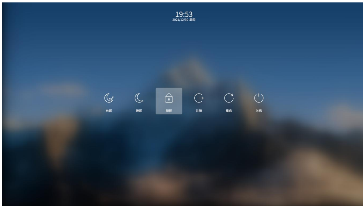
图 1.5 电源
