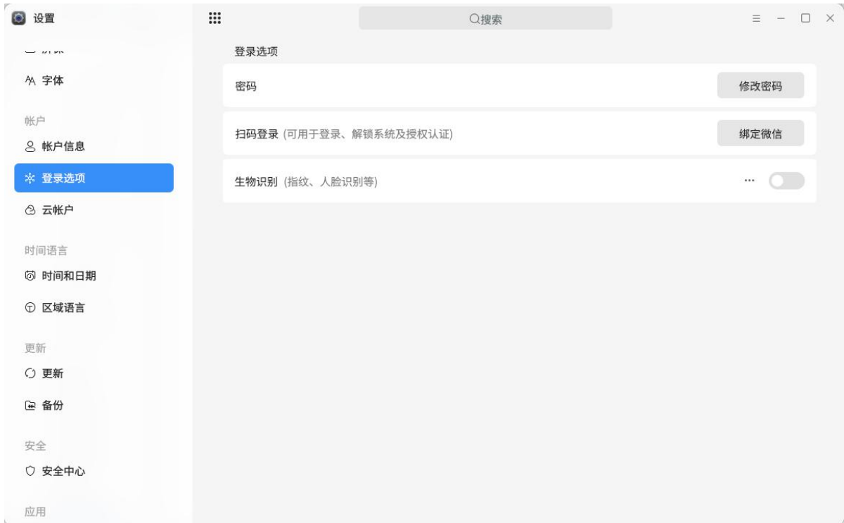
图 2.136 登录选项
