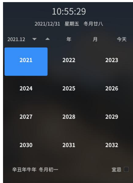
图 1.15 年份切换
