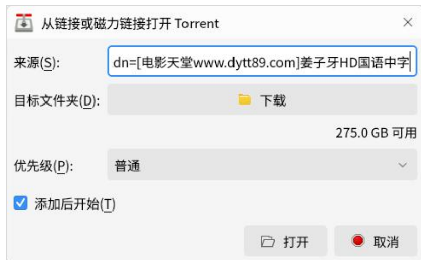
图 3.208 打开链接
