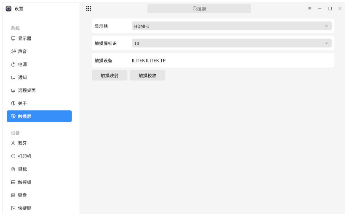
图 2.11 触摸屏
