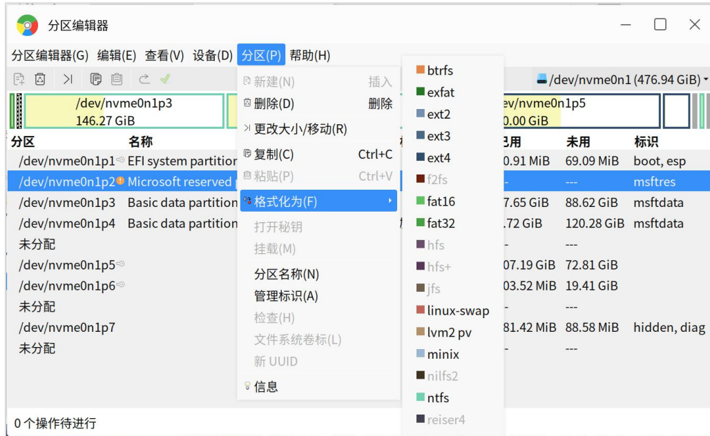
图 5.52 格式化分区
