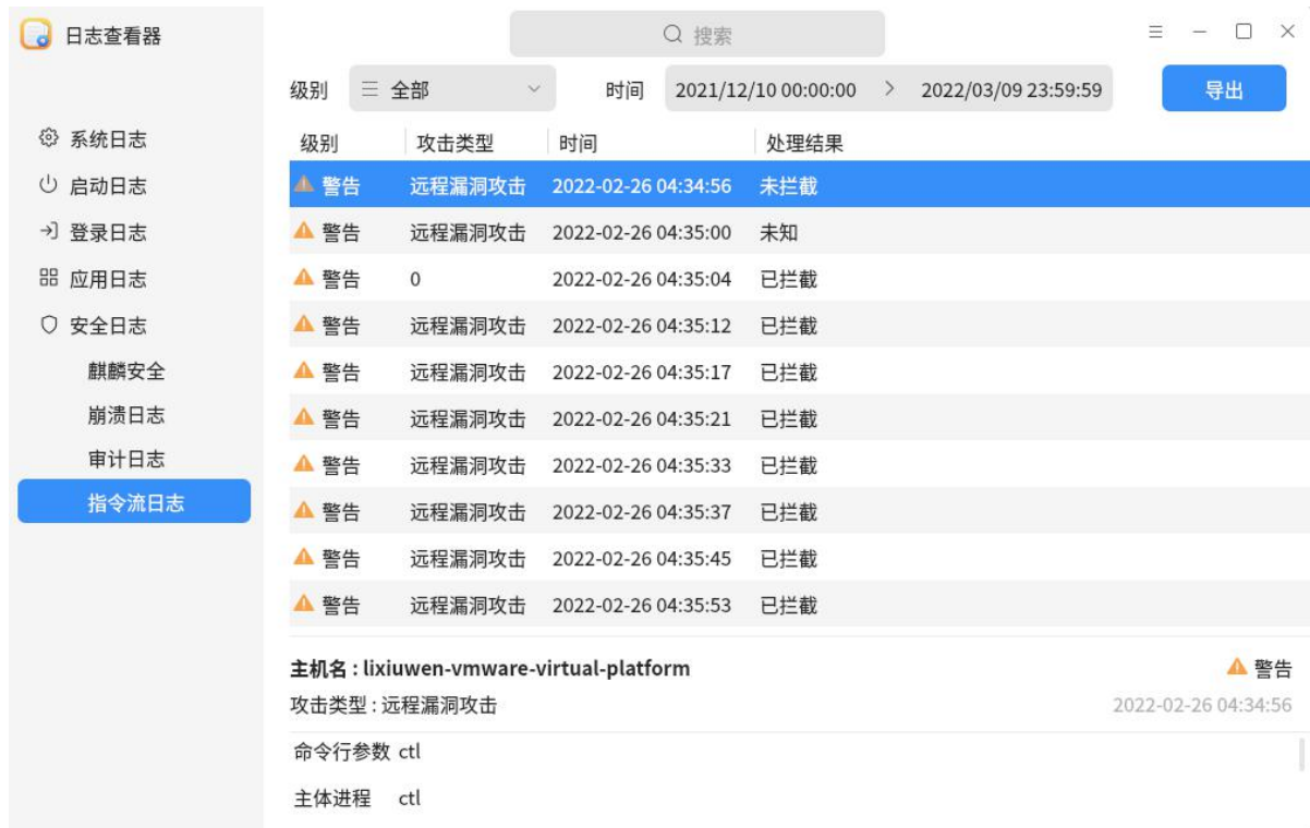
图 5.16 指令流日志
