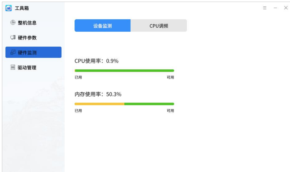
图 5.44 硬件监测
