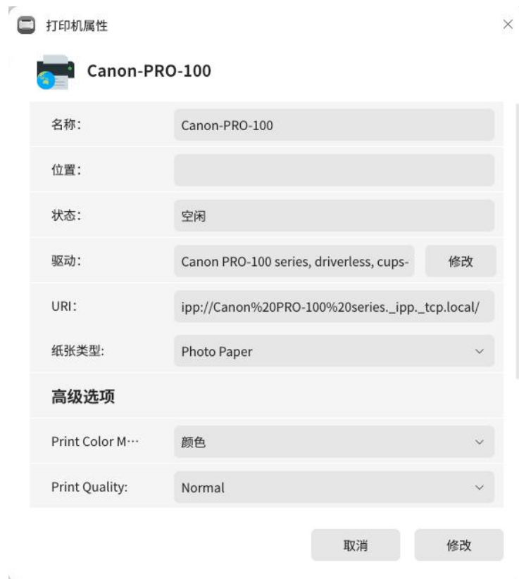
图 3.59 打印机属性
