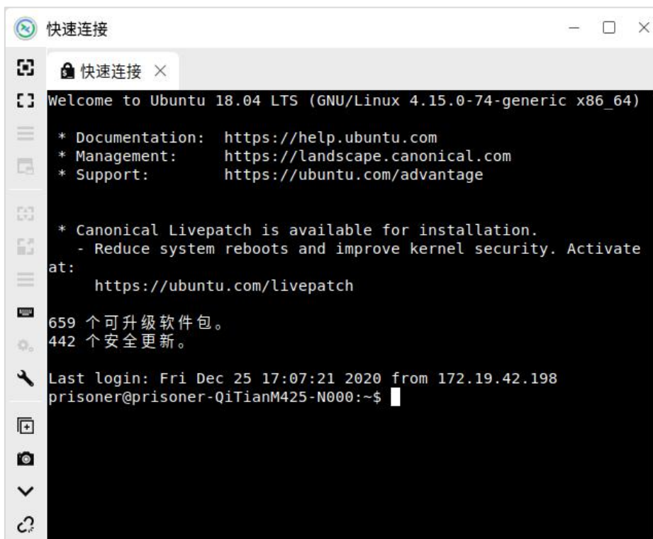
图 3.202 连接成功
