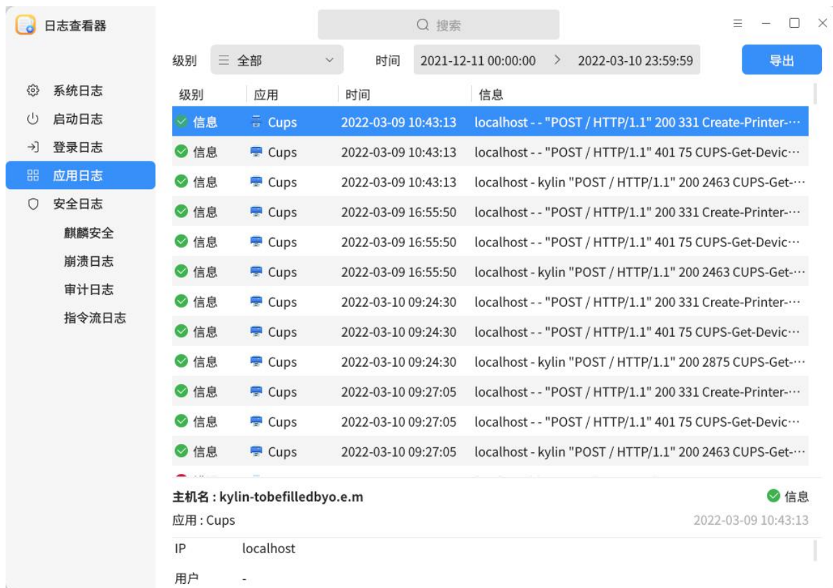
图 5.12 应用日志
