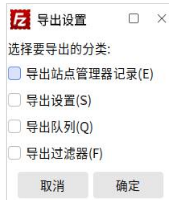
图 3.191 导出设置
