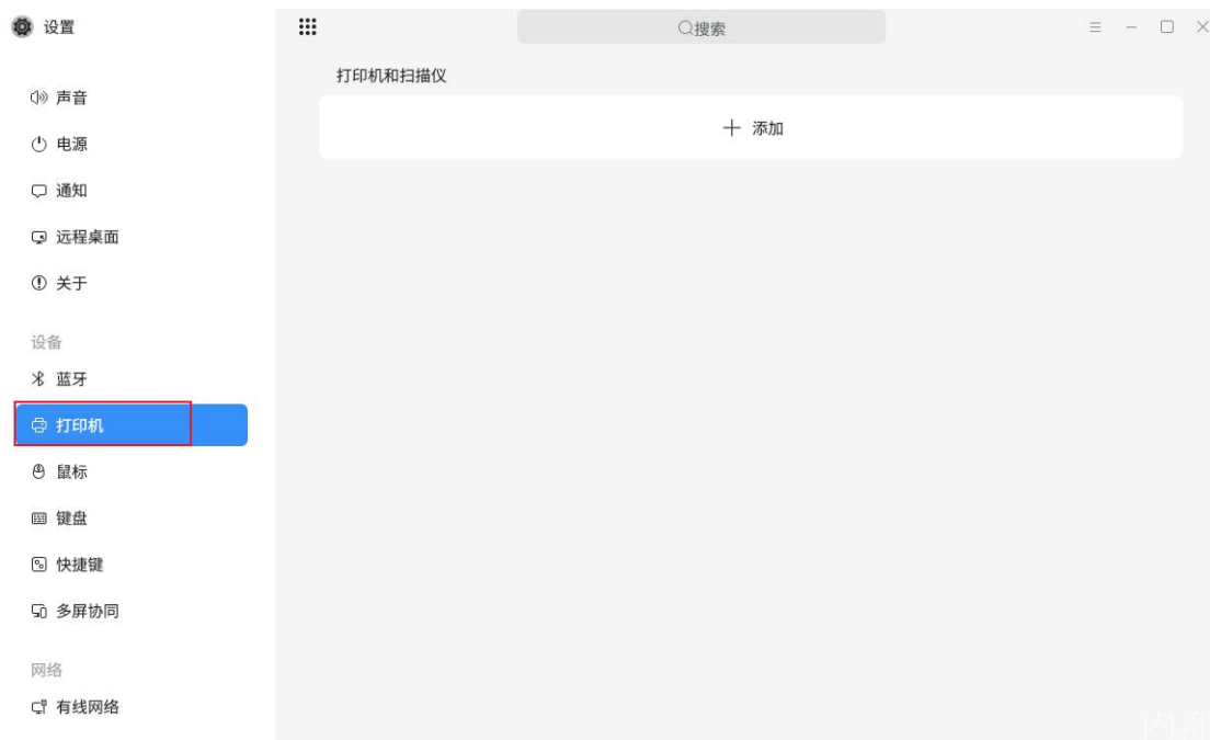
图 2.30 打印机
