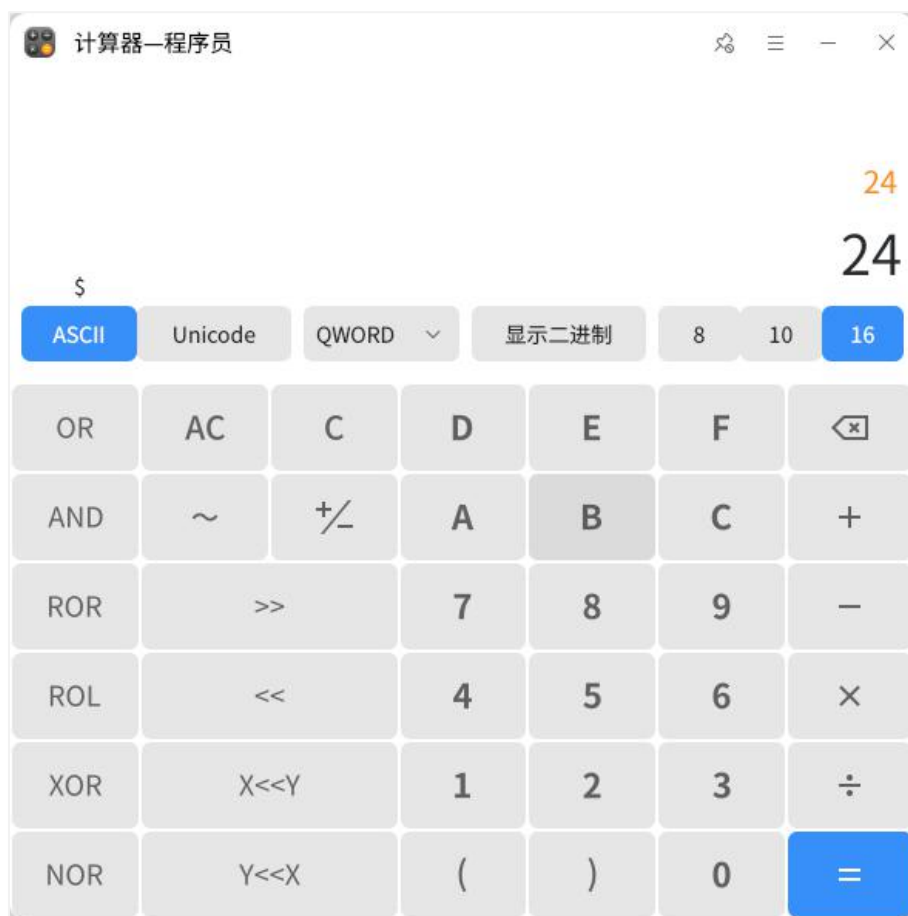
图 3.106 程序员计算
