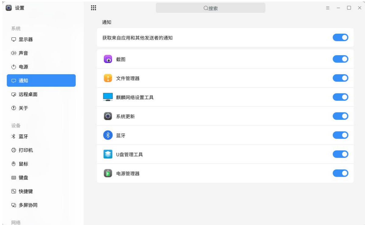
图 2.6 通知
