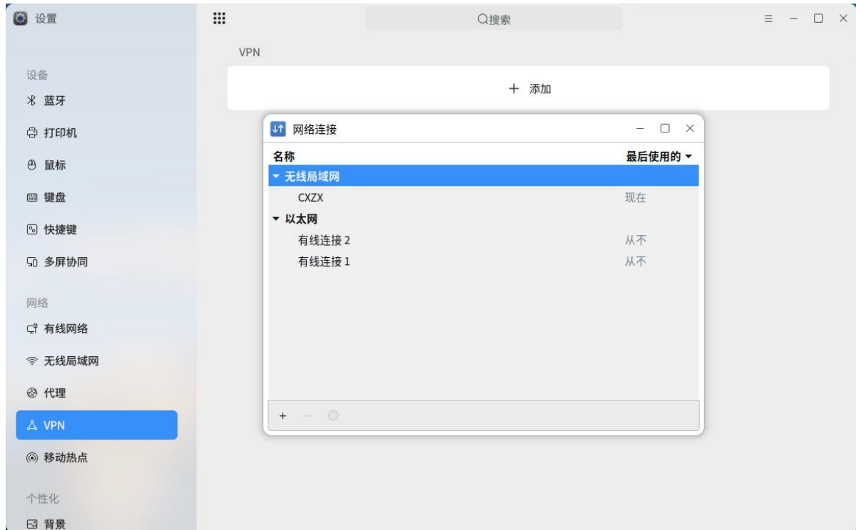
图 2.121 VPN 设置
