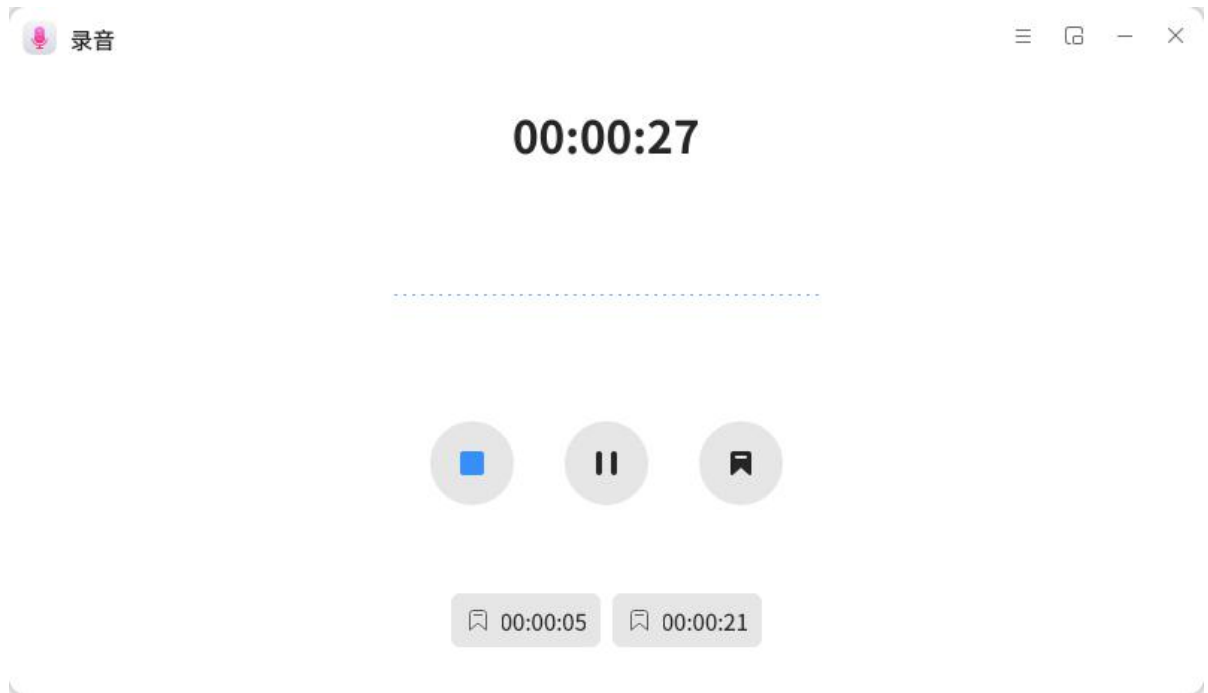
图 3.49 音频录制
