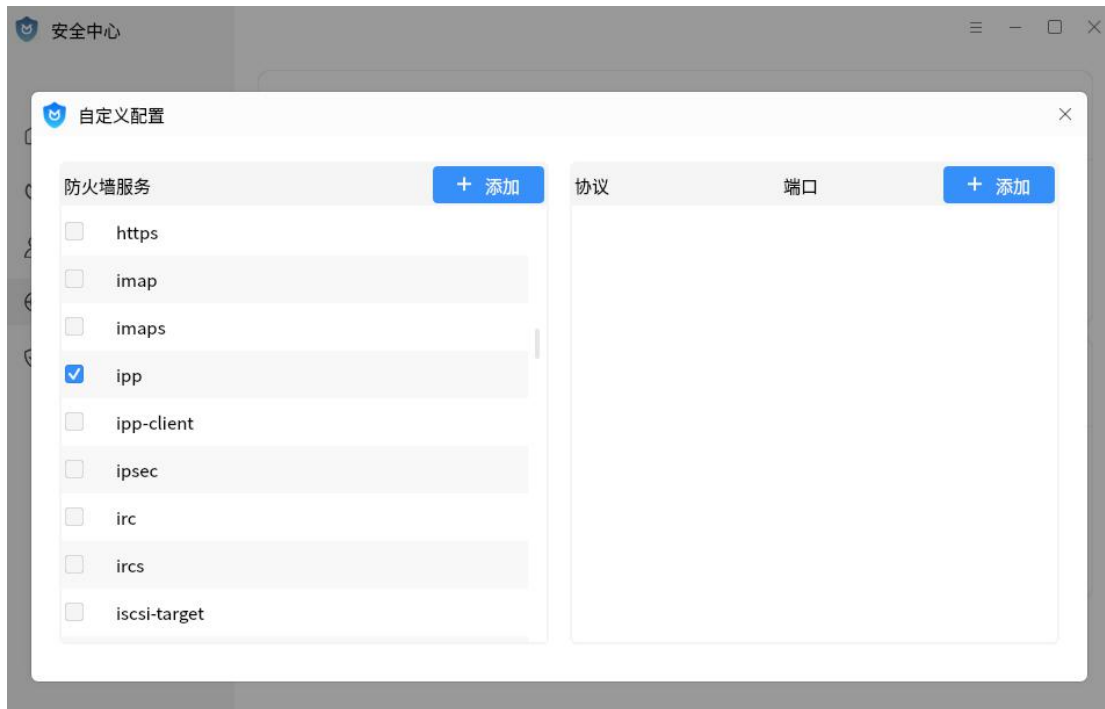
图 2.35 自定义配置
