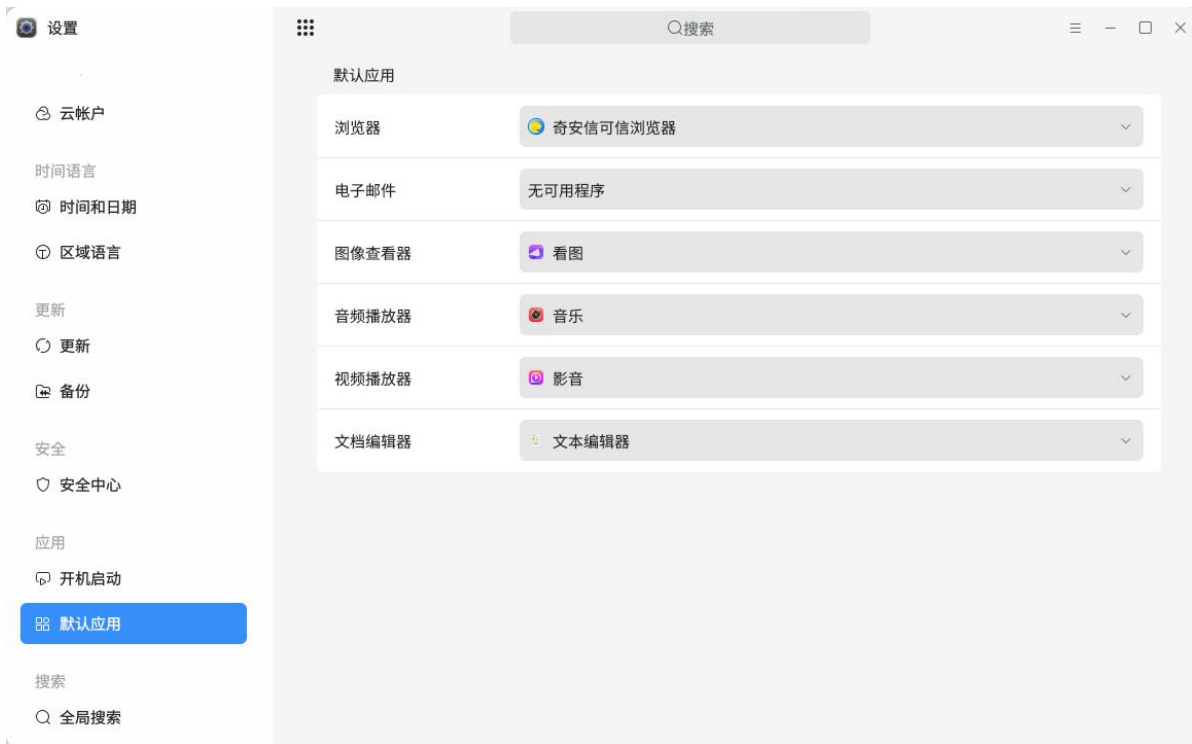
图 2.149 默认应用
