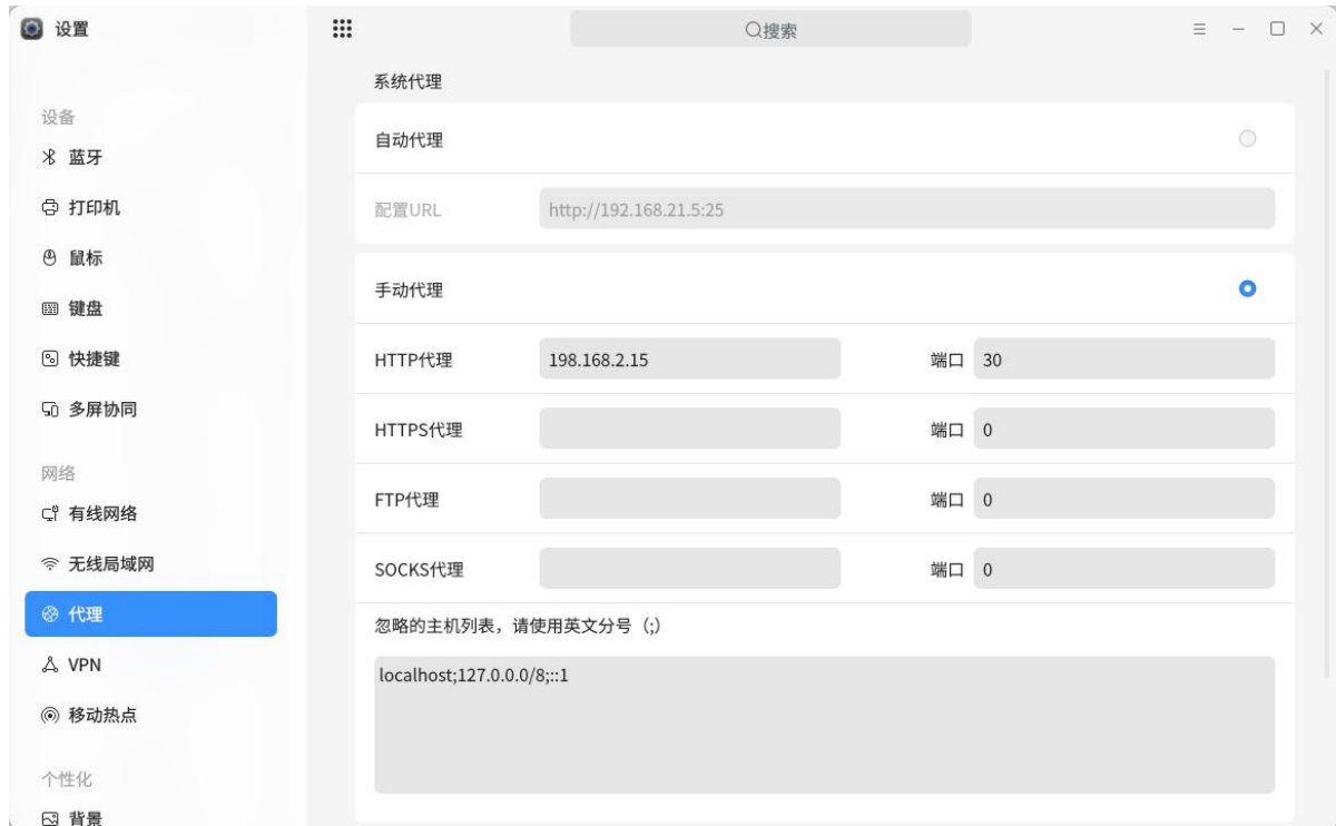
图 2.119 手动代理
