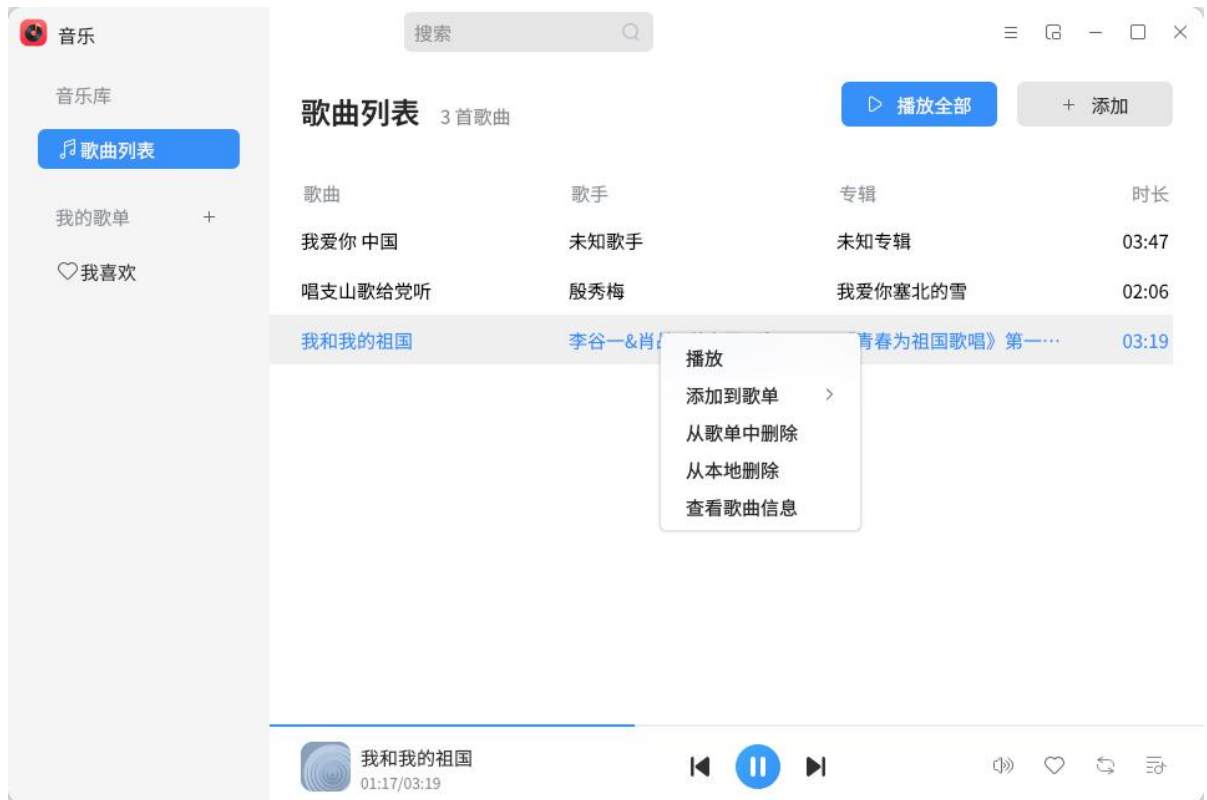
图 3.138 歌曲设置
