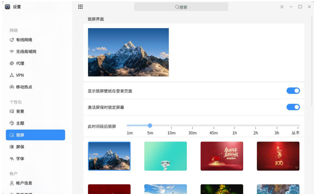
图 2.125 设置锁屏
