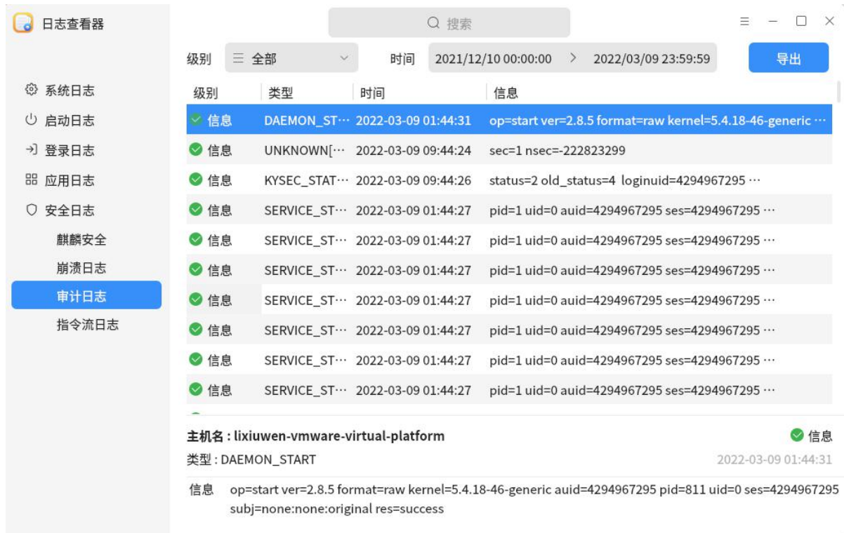
图 5.15 审计日志
