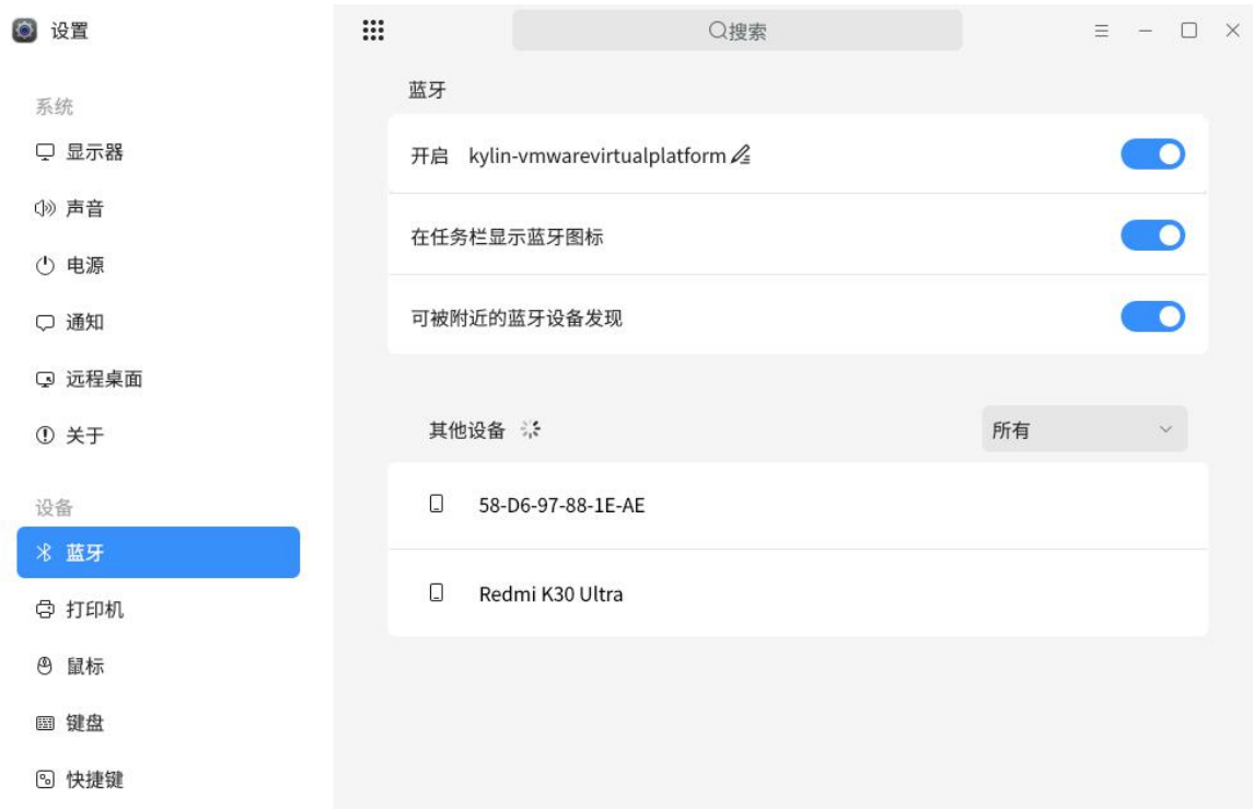
图 2.12 蓝牙
