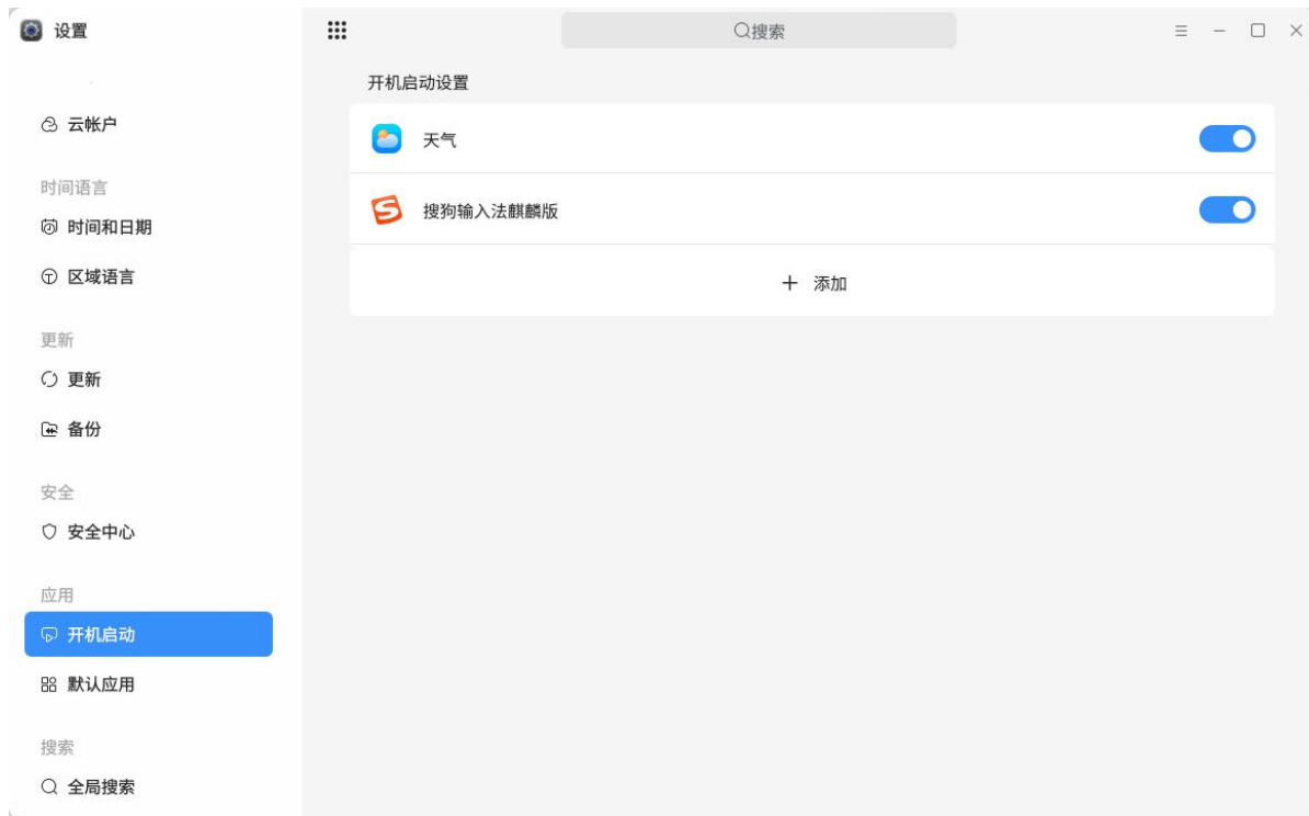
图 2.148 开机启动
