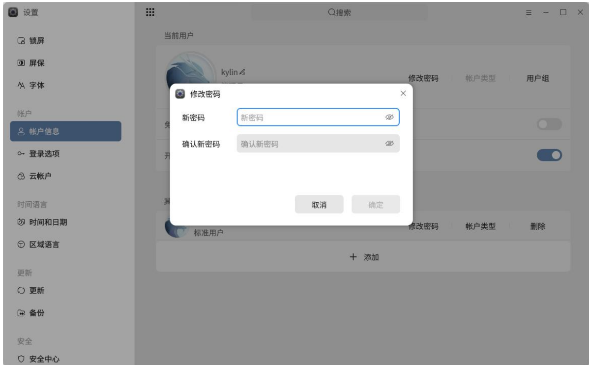
图 2.133 修改密码
