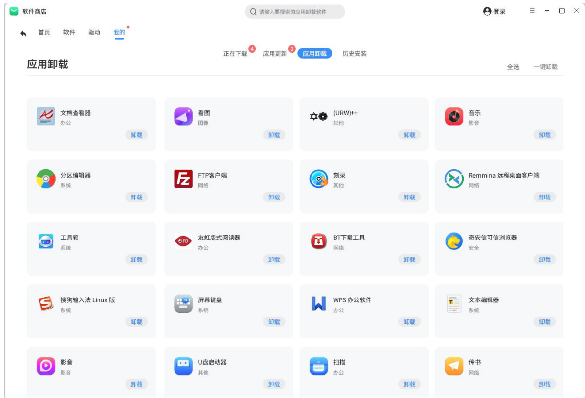
图 3.21 应用卸载
