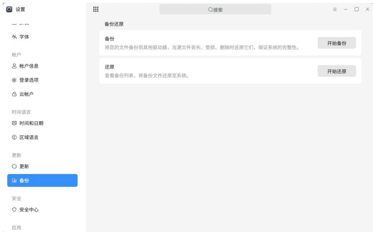
图 2.146 备份还原
