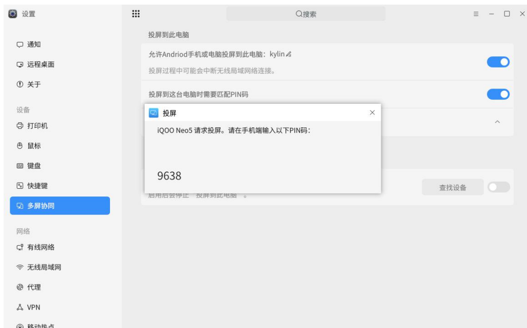
图 2.73 电脑端
