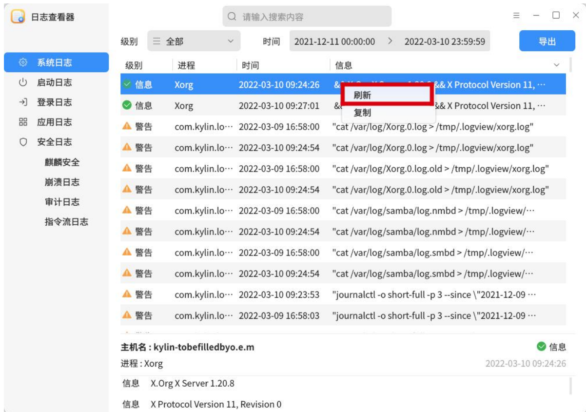
图 5.22 刷新日志
