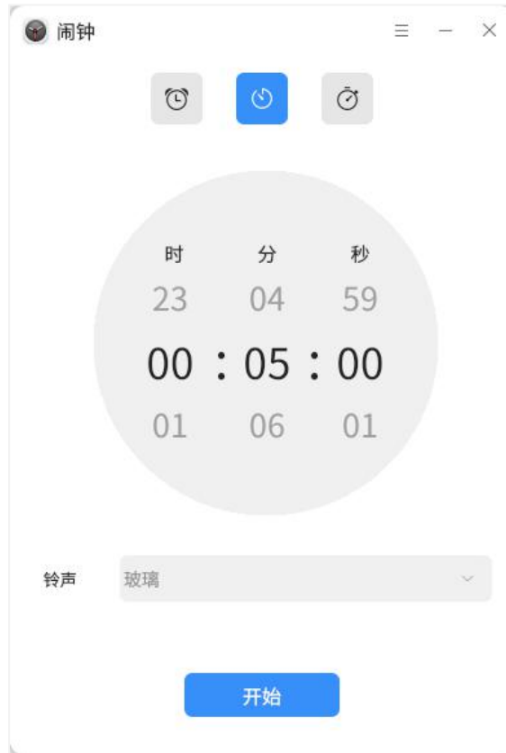
图 3.87 倒计时
