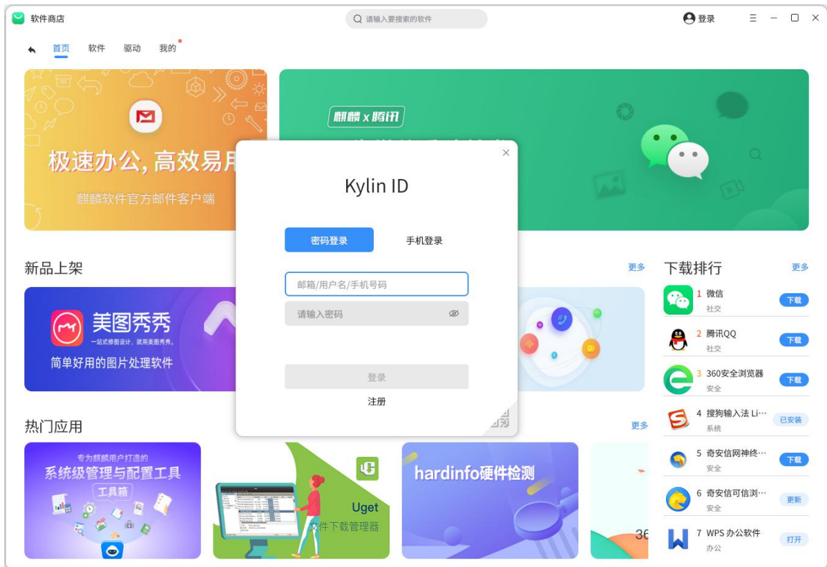
图 3.12 密码登录
