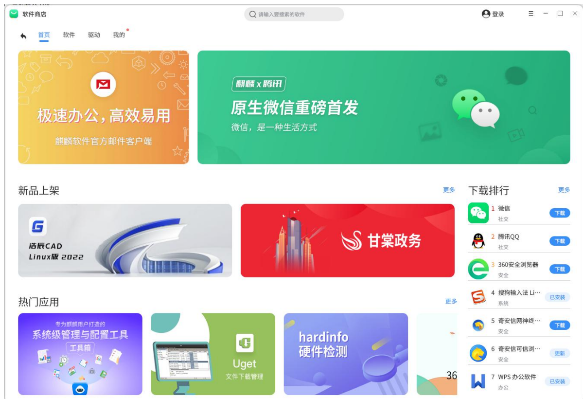
图 3.14 首页
