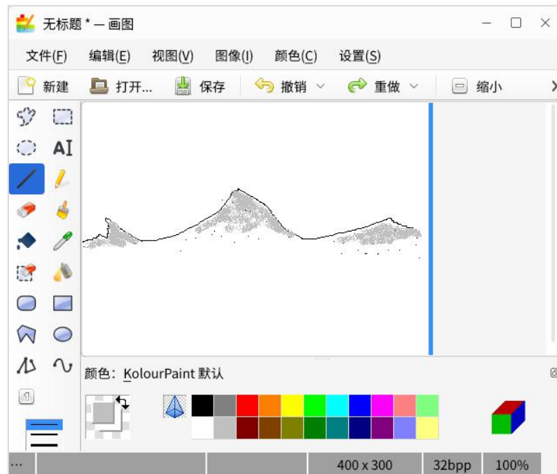
图 3.131 画图
