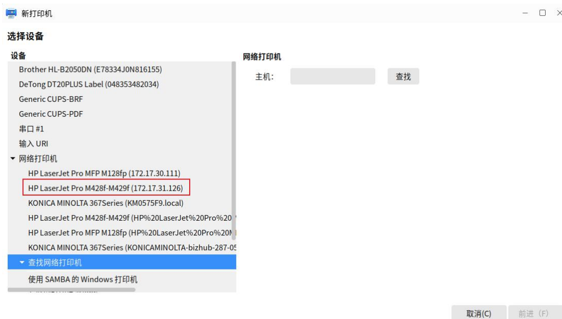
图 2.24 添加打印机
