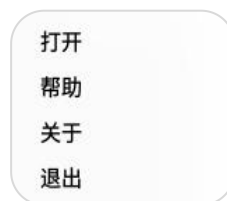
图 3.127 看图菜单栏
