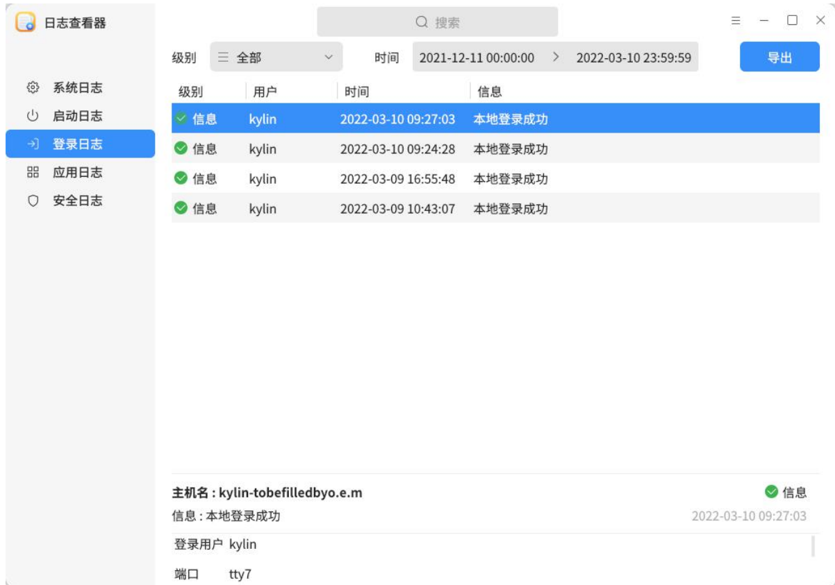
图 5.11 登录日志
