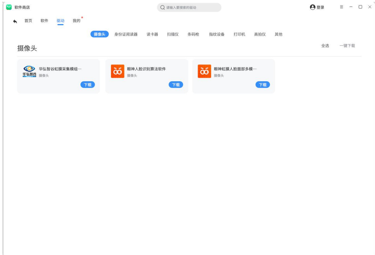
图 3.16 驱动页面
