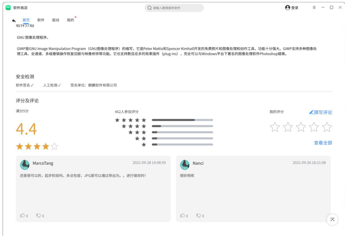
图 3.24 软件评价
