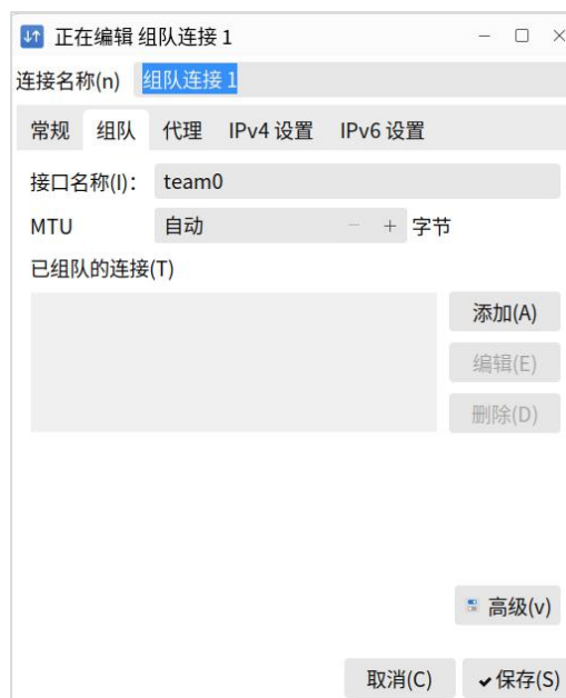
图 2.103 编辑组队
