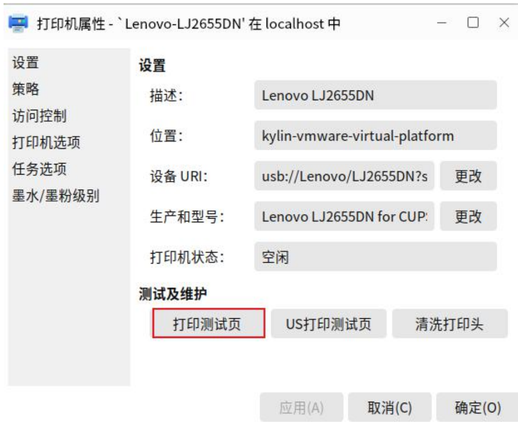
图 2.21 打印测试页
