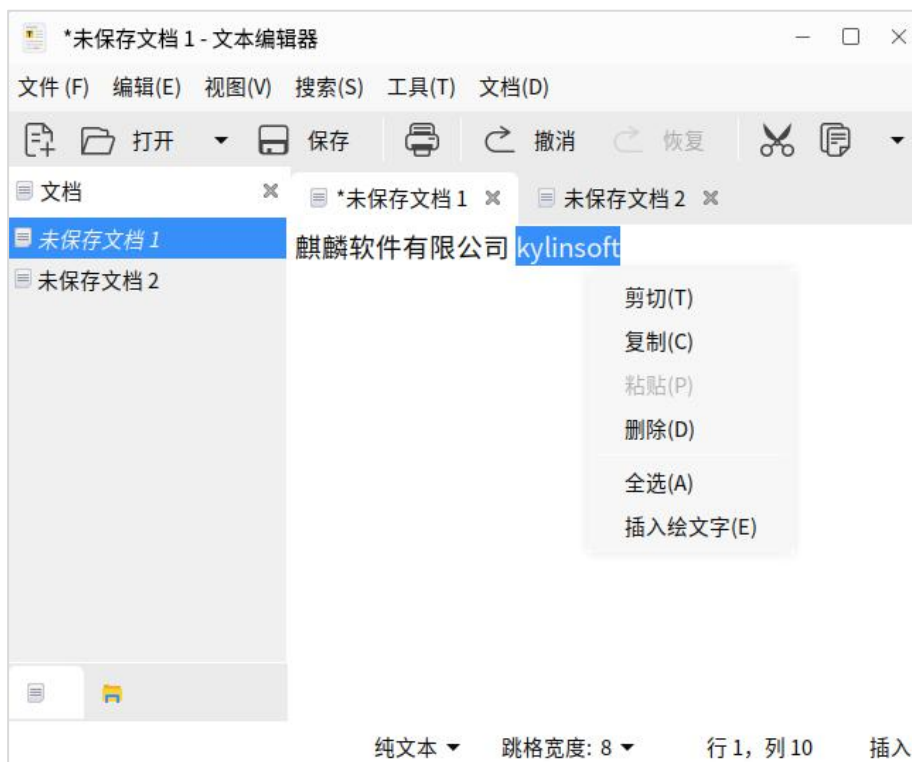
图 3.33 文本编辑器
