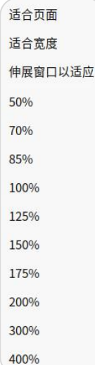
图 3.38 查看文档
