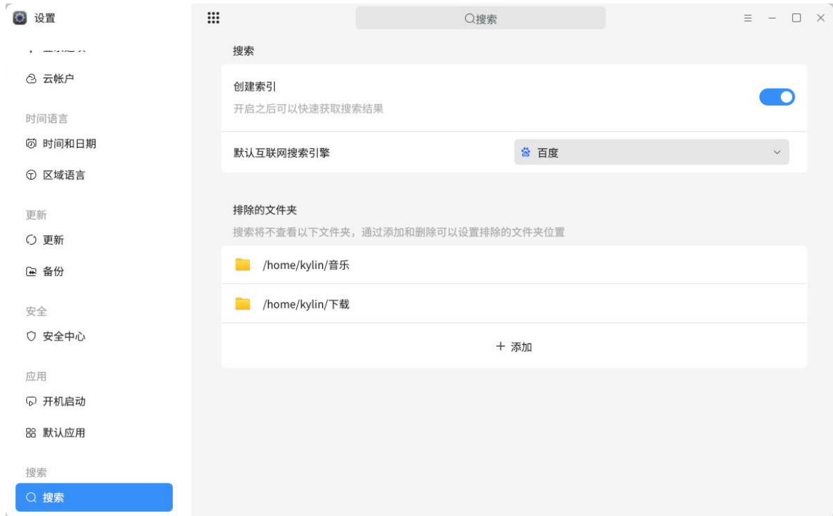
图 2.154 搜索设置
