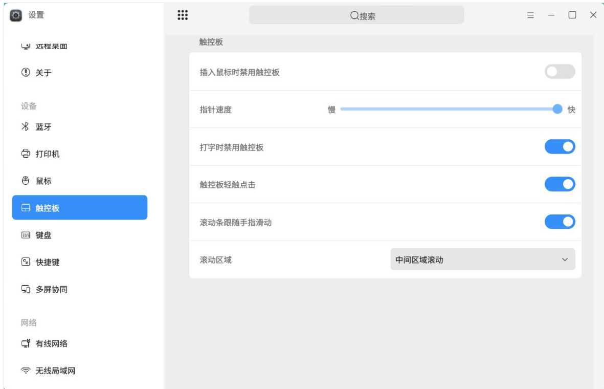
图 2.67 触控板
