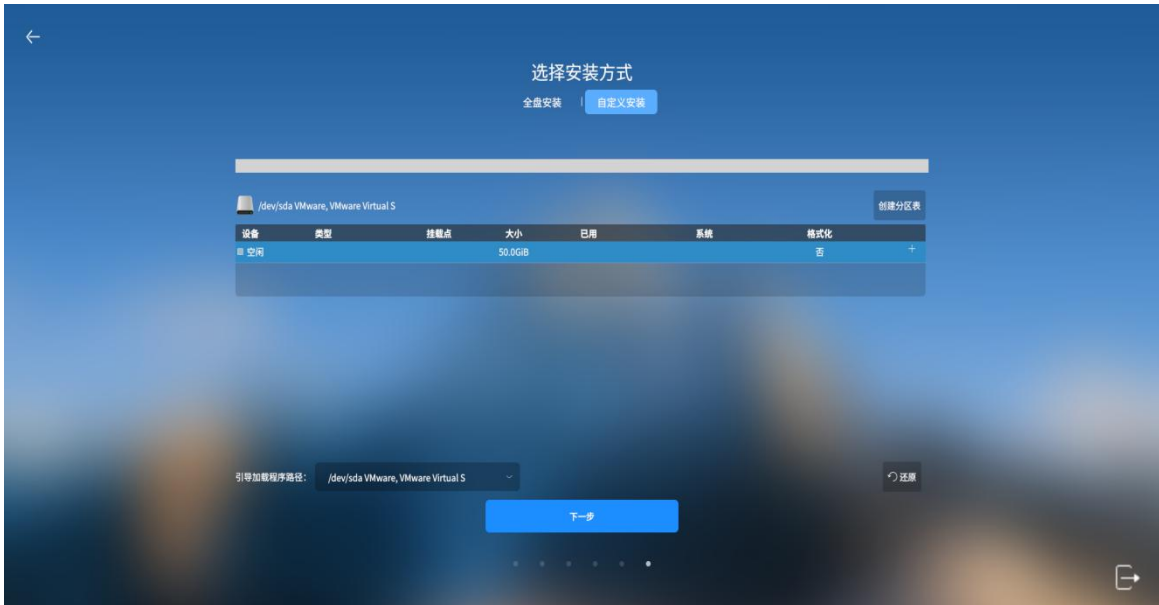
图 14 自定义安装
