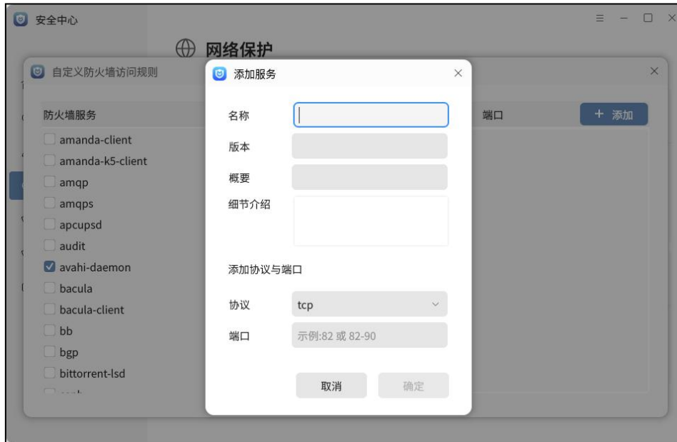
图 4.29 添加服务
