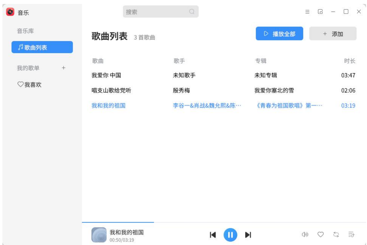
图 3.137 歌曲列表
