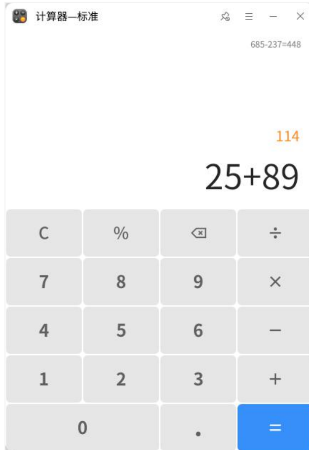
图 3.103 标准计算
