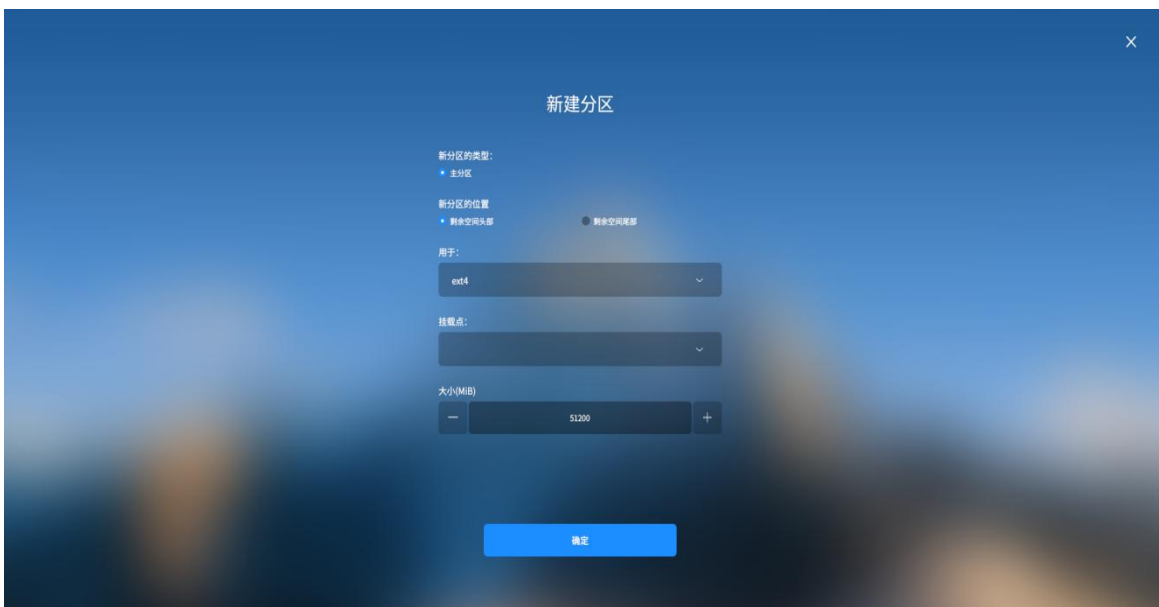
图 15 创建分区
