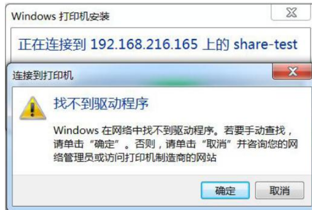
图 2.45 连接提示
