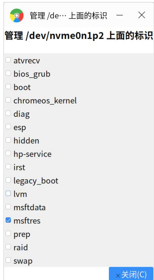
图 5.53 标识管理
