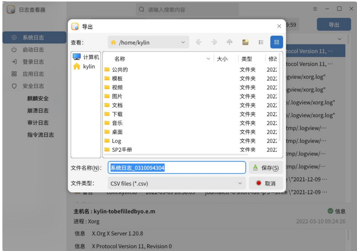
图 5.21 导出文件
