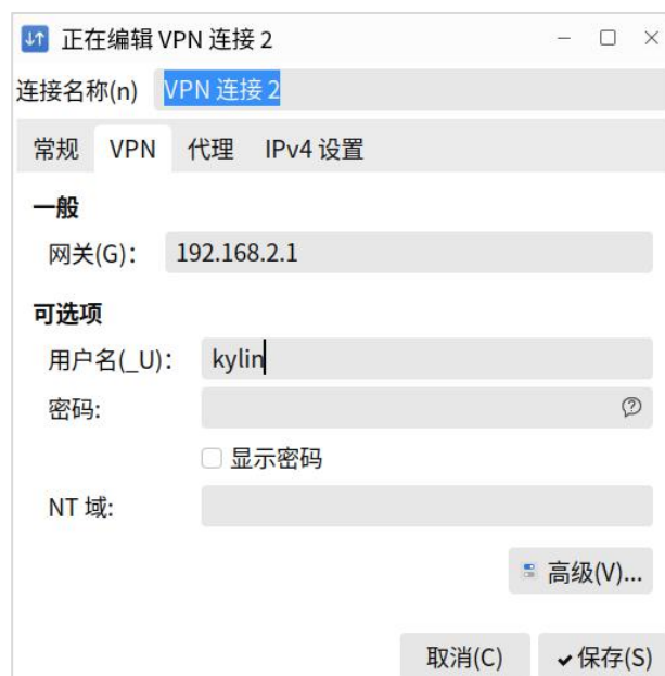
图 2.114 编辑 VPN
