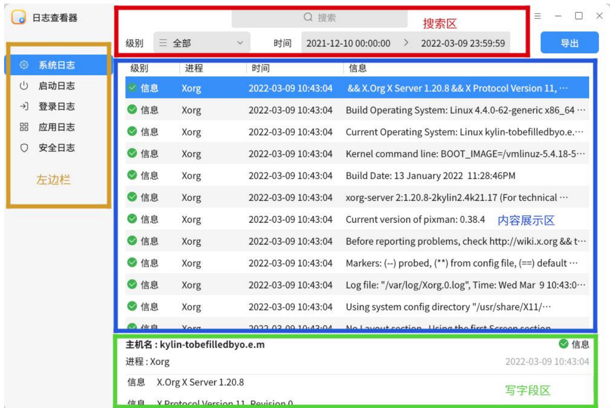
图 5.2 区域介绍
