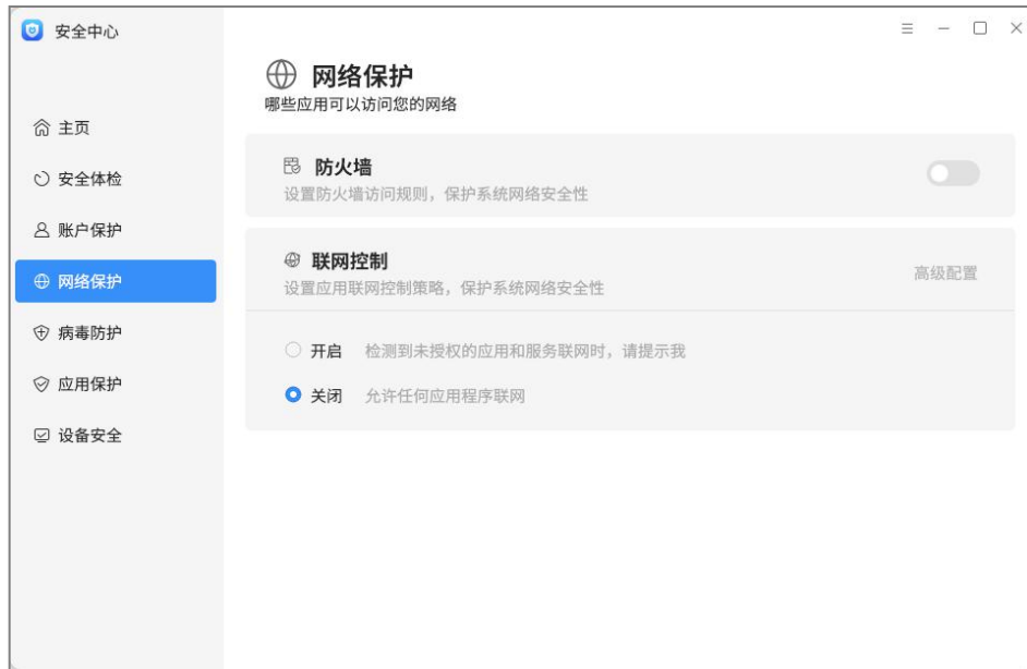
图 4.27 关闭防火墙
