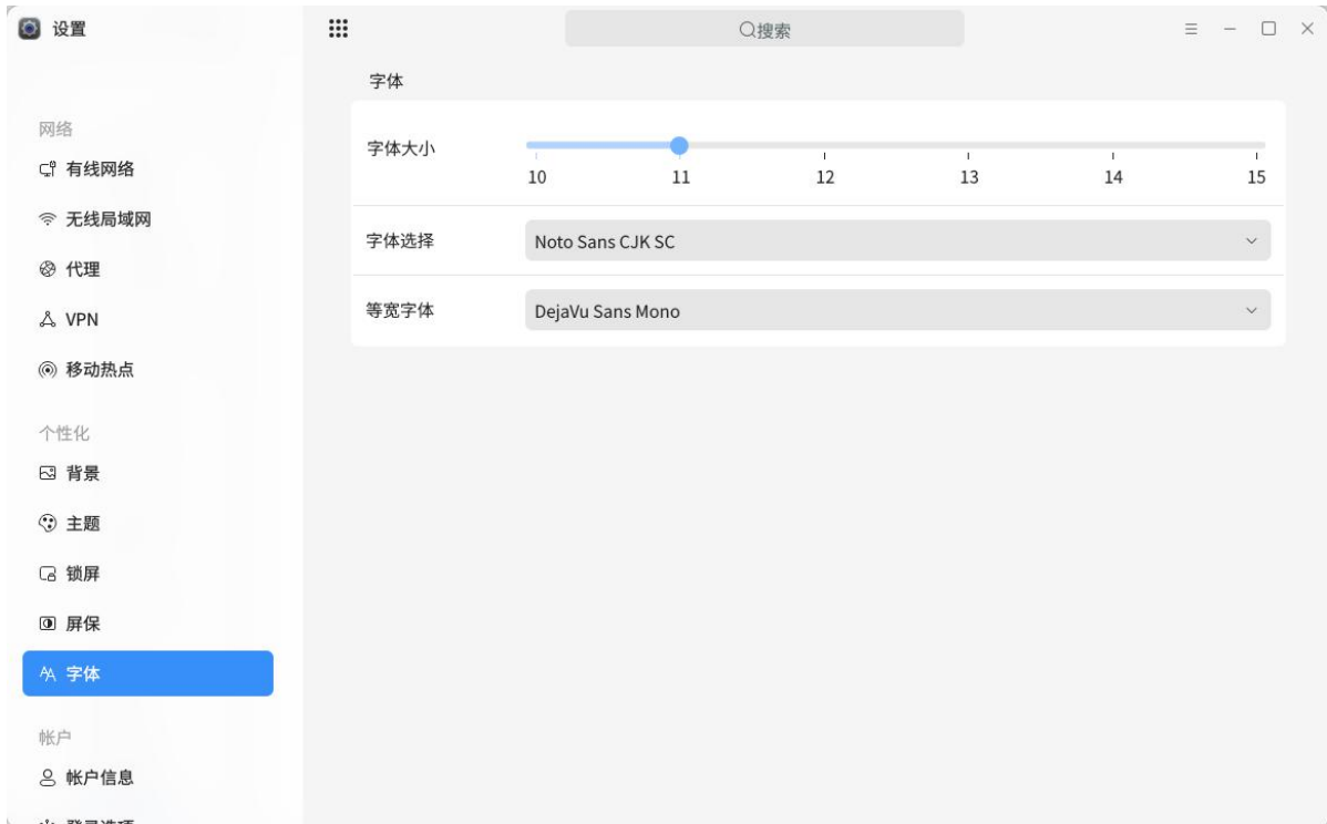
图 2.128 设置字体
