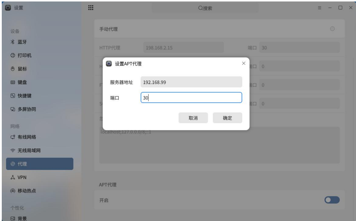
图 2.120 APT 代理
