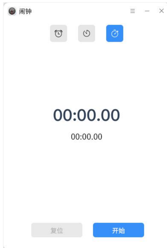
图 3.96 秒表
