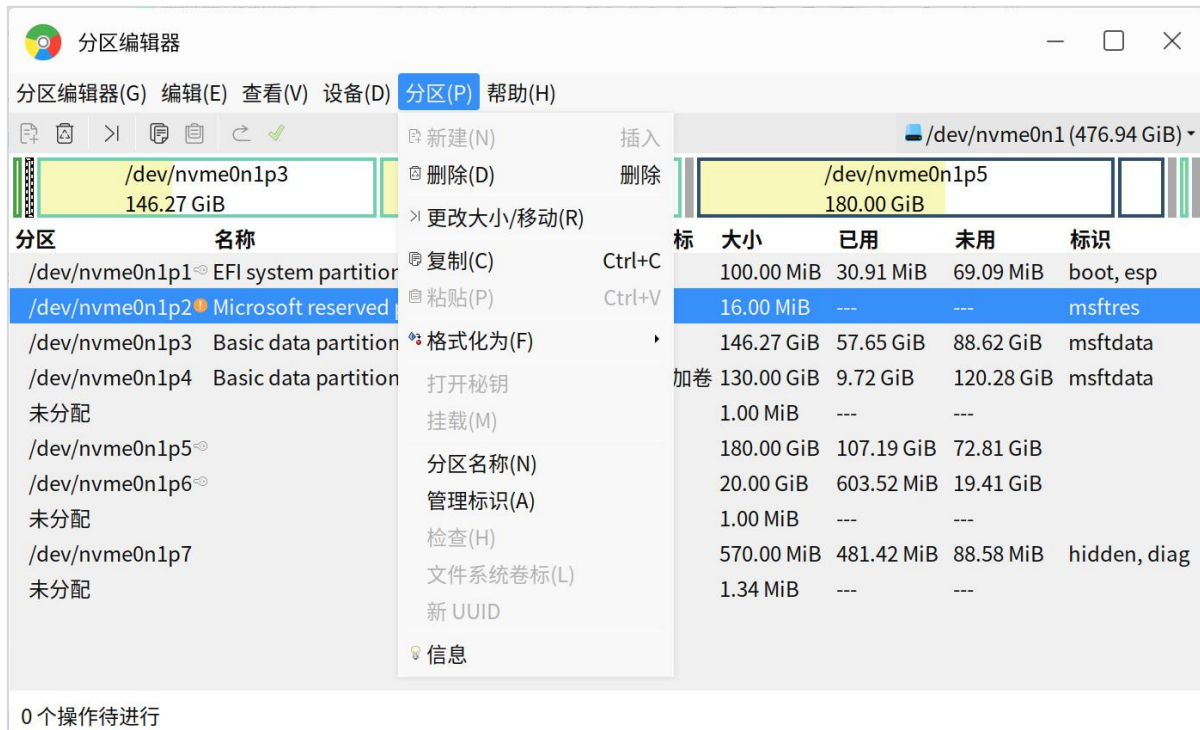
图 5.49 分区菜单
