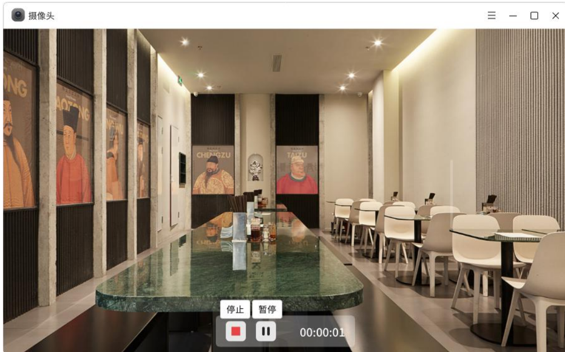
图 3.81 录像模式
