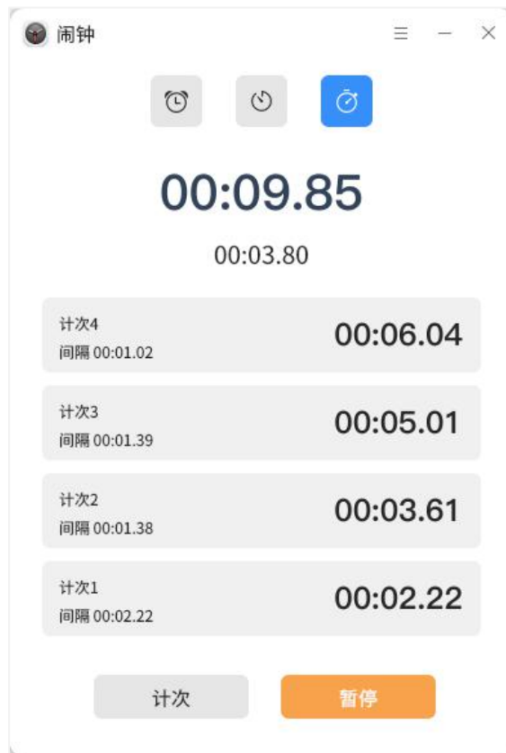
图 3.97 计时和计次
