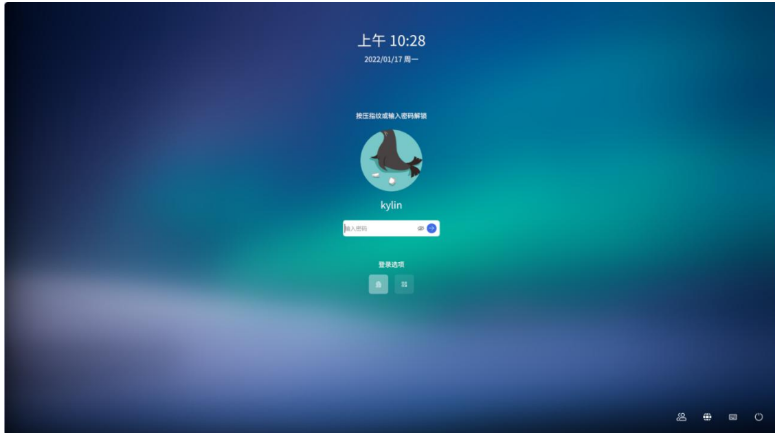
图 5.66 登陆
