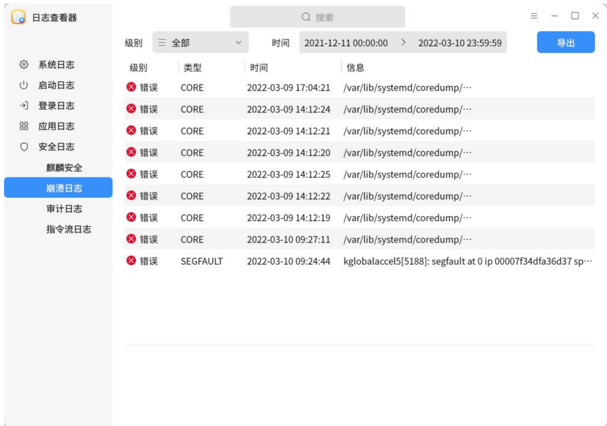
图 5.14 崩溃日志
