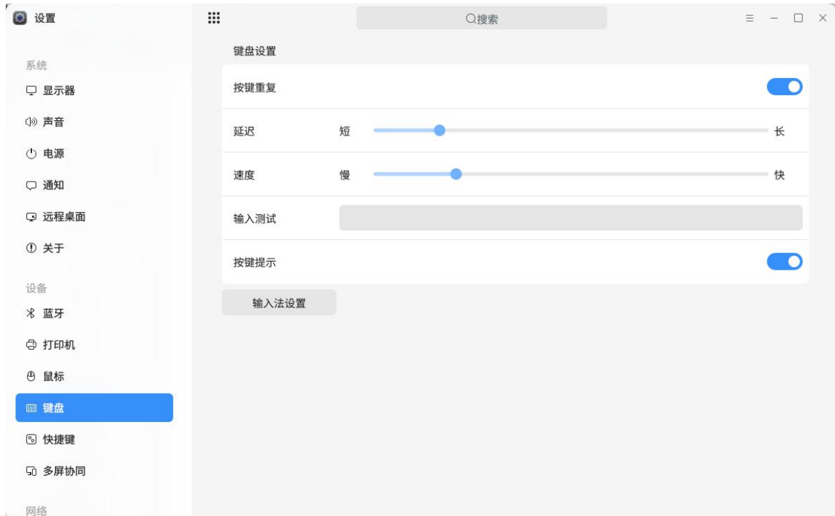
图 2.68 键盘设置
