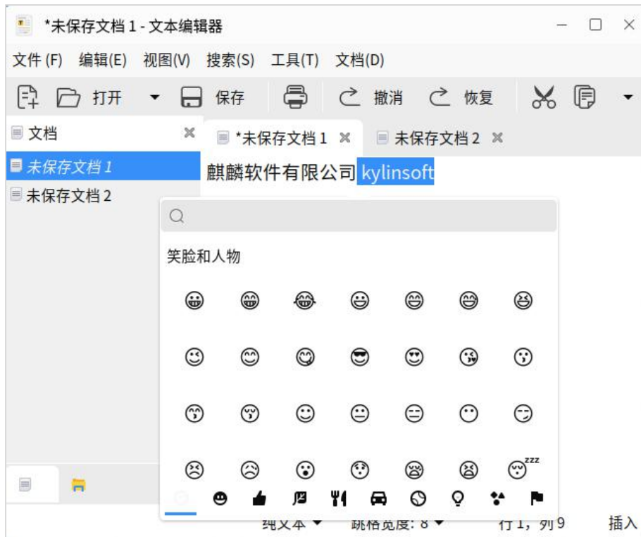
图 3.34 插入绘文字
