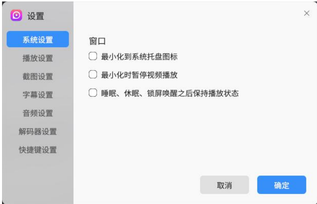
图 3.152 影音设置
