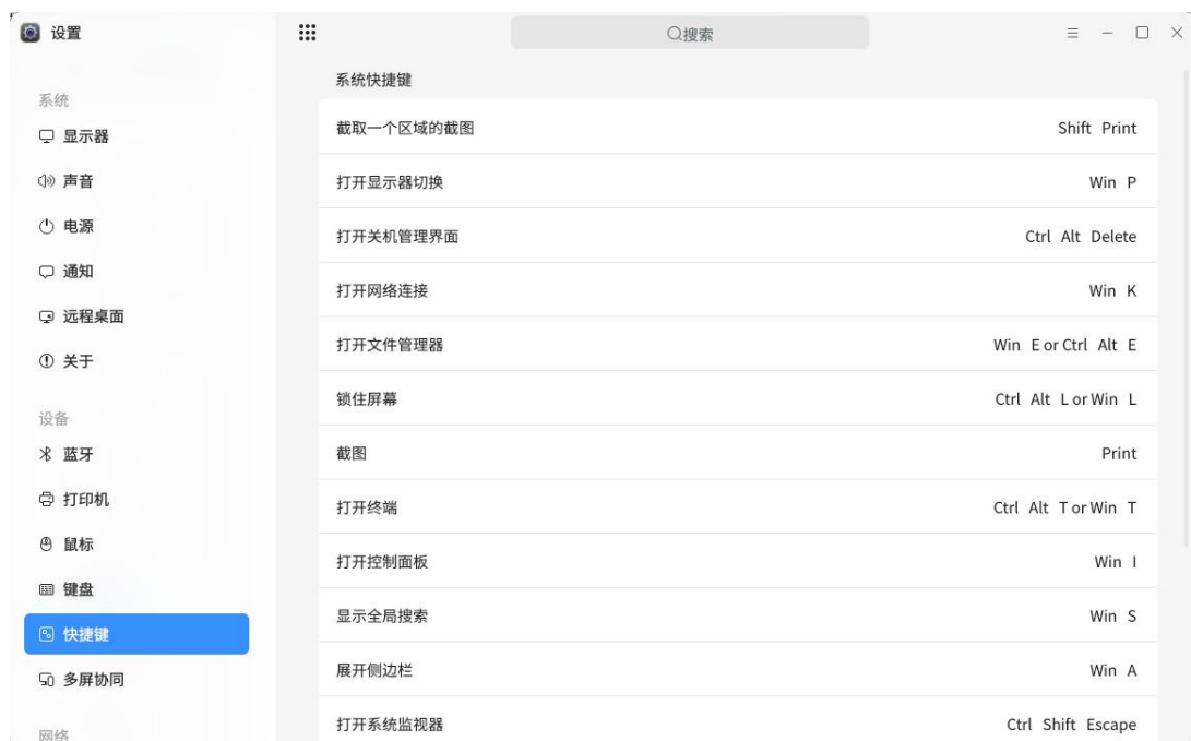
图 2.70 系统快捷键
