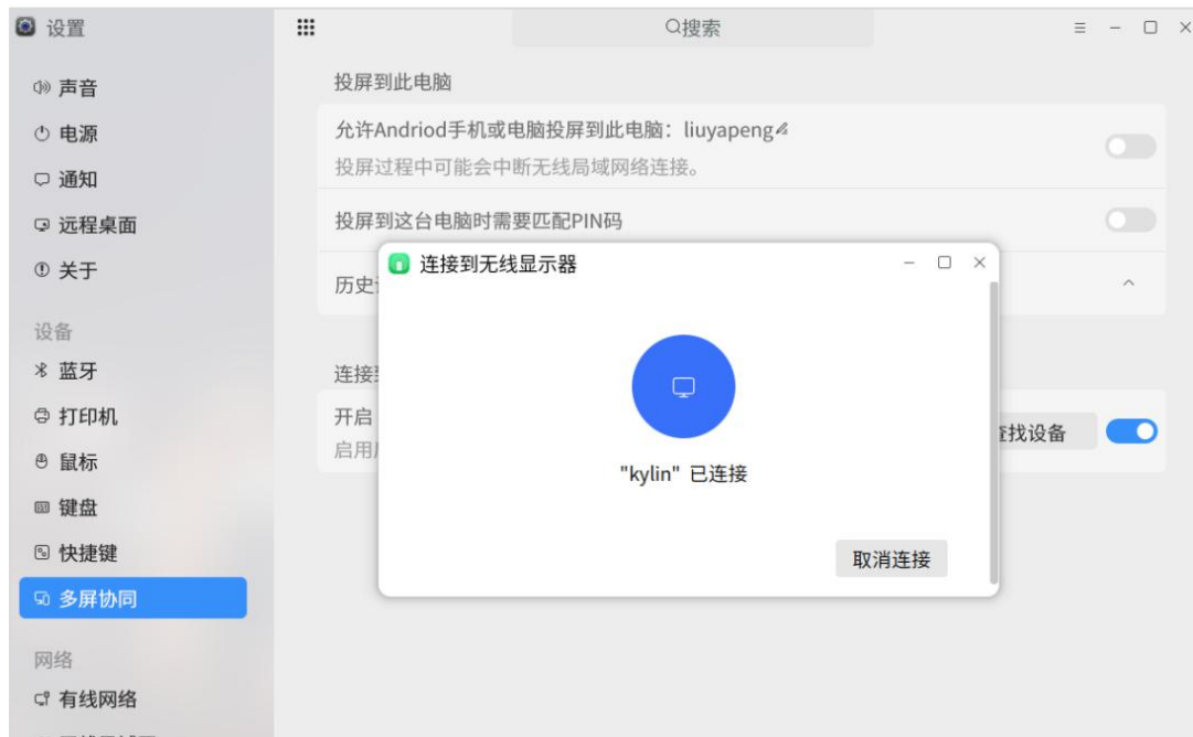
图 2.79 连接成功
