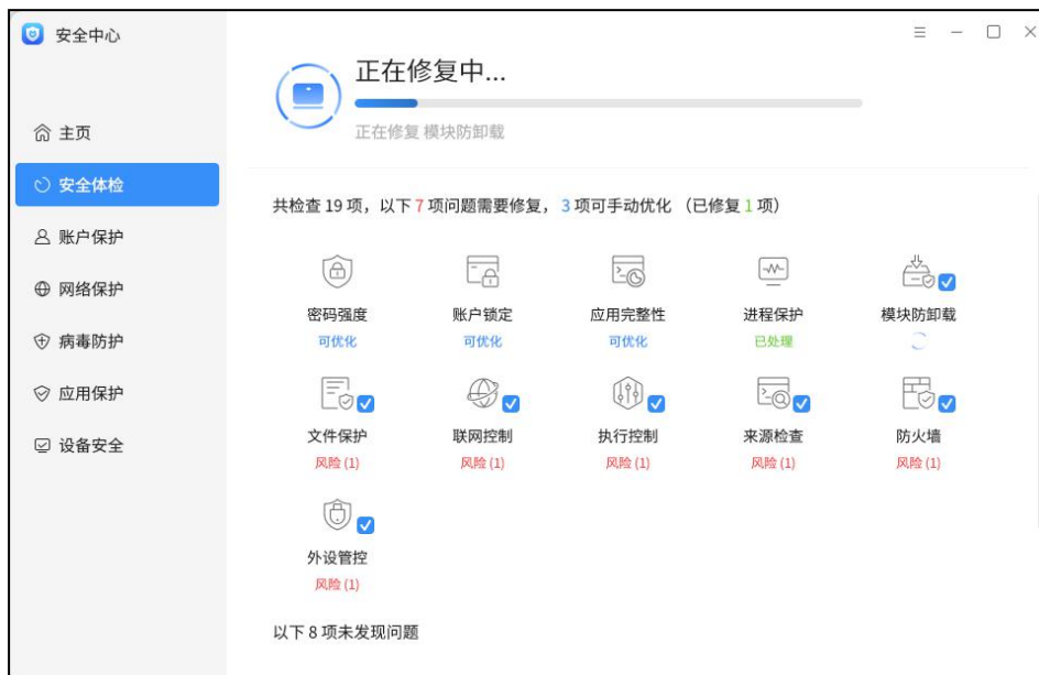
图 4.19 一键修复中
