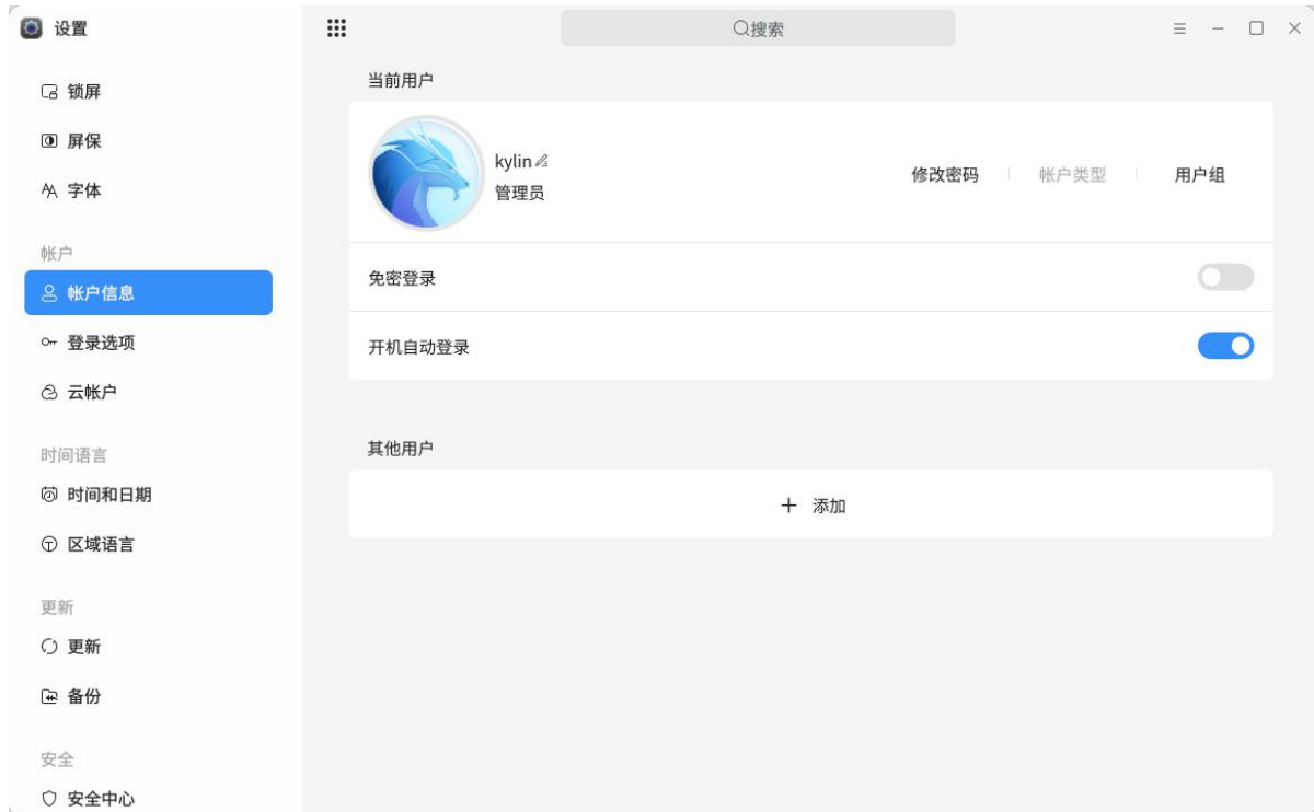
图 2.129 账户信息
