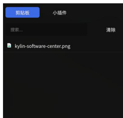
图 1.10 剪切板
