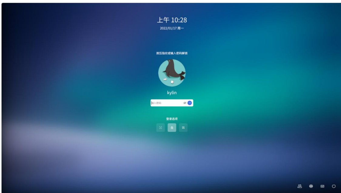
图 5.67 选择设备
