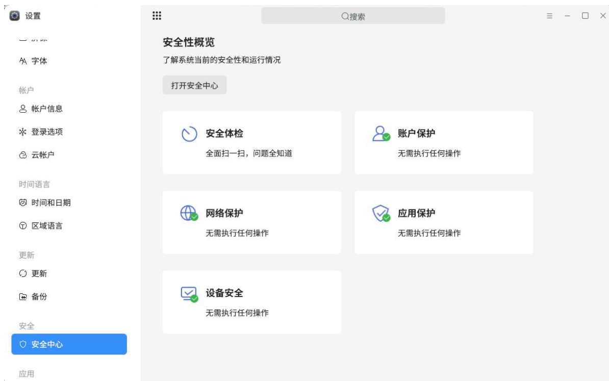
图 2.147 安全中心
