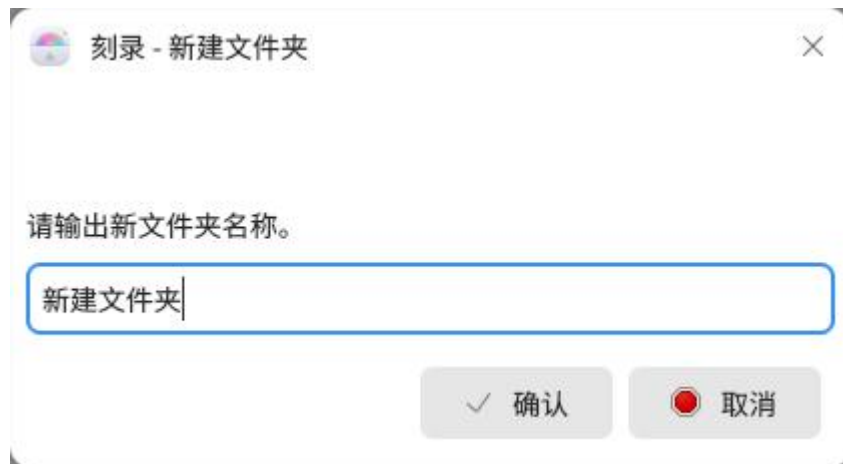
图 3.167 新建文件夹
