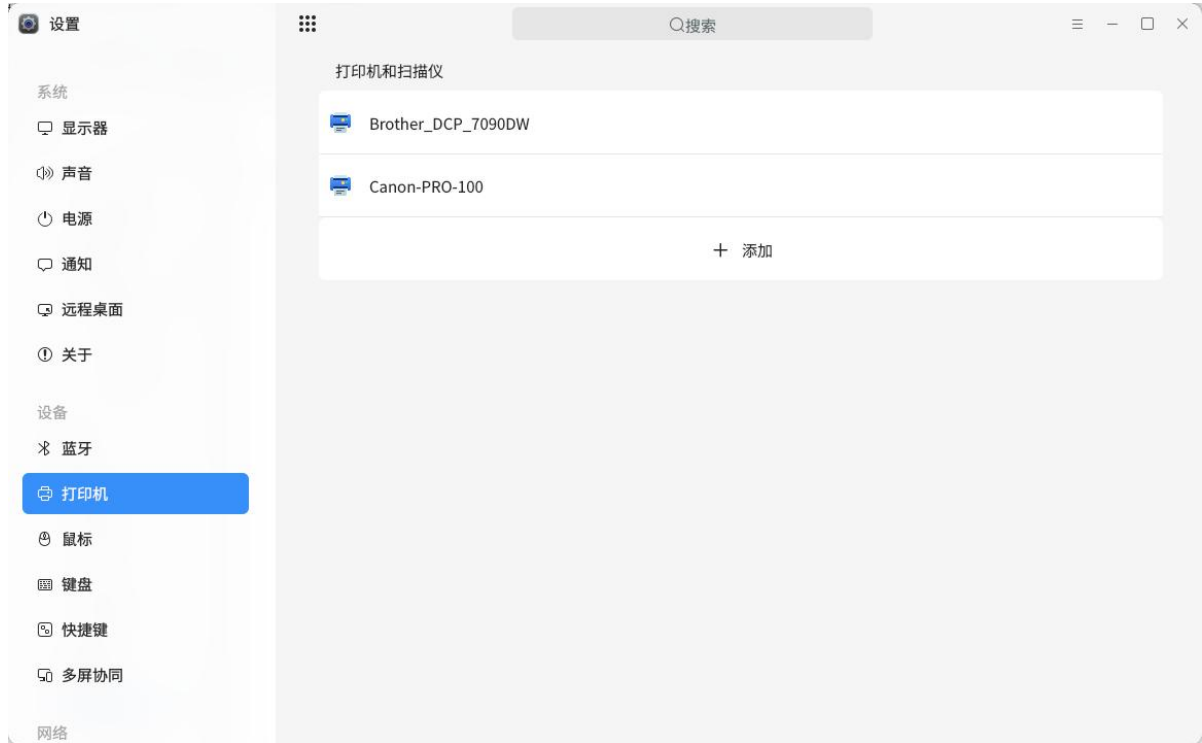
图 2.14 打印机
