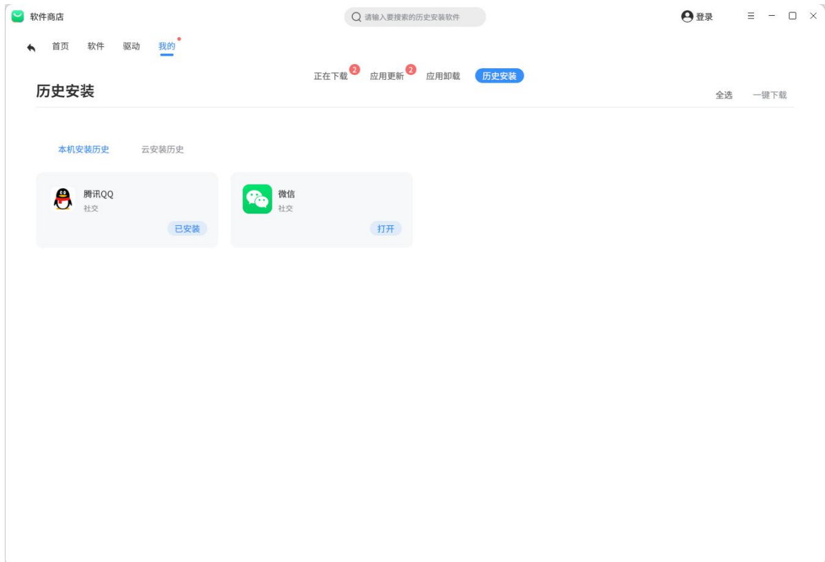
图 3.22 历史安装
