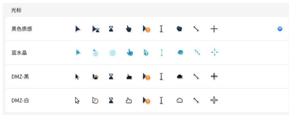
图 2.66 光标主题
