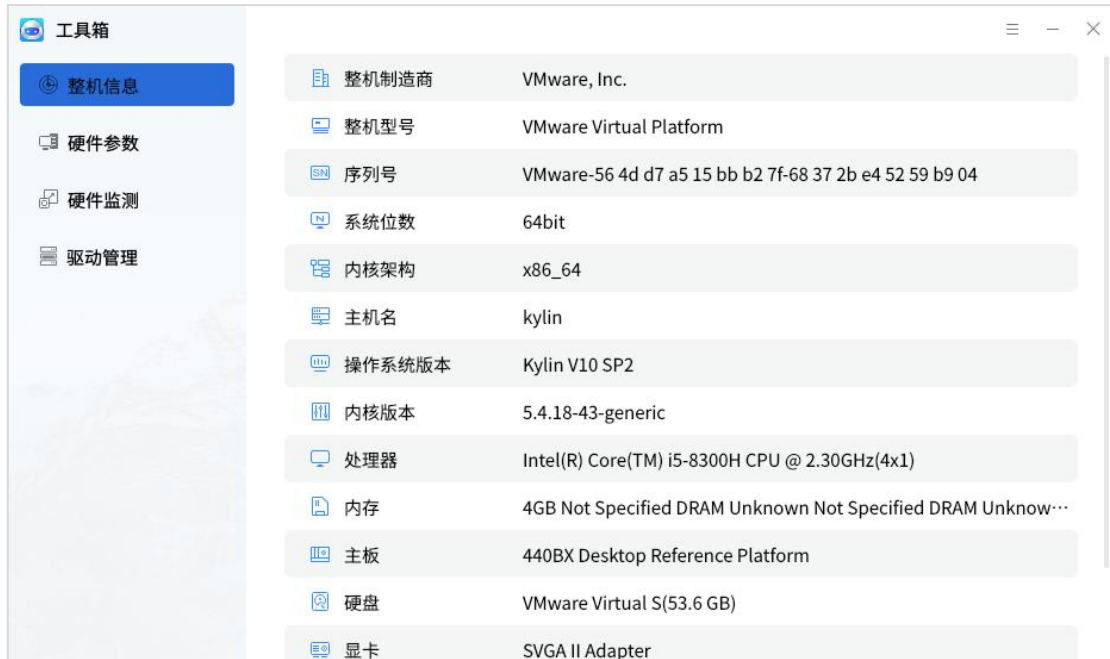
图 5.42 整机信息
