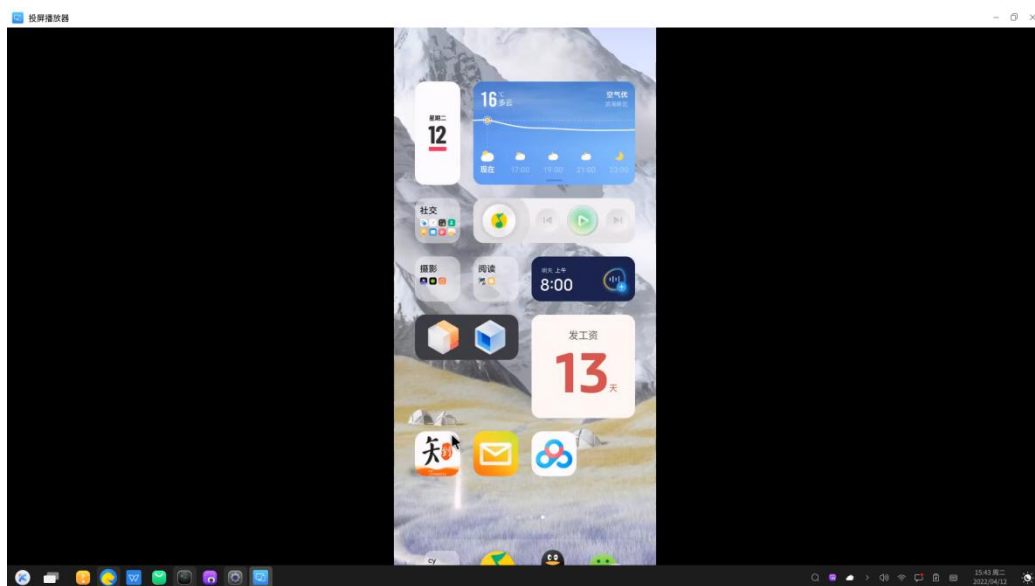
图 2.75 效果展示
