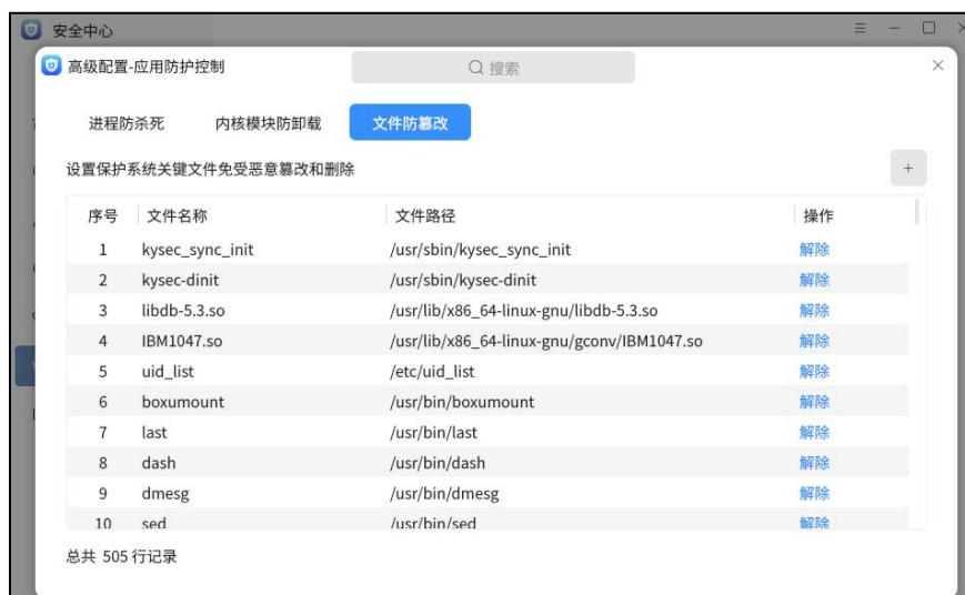
图 4.46 文件防篡改
