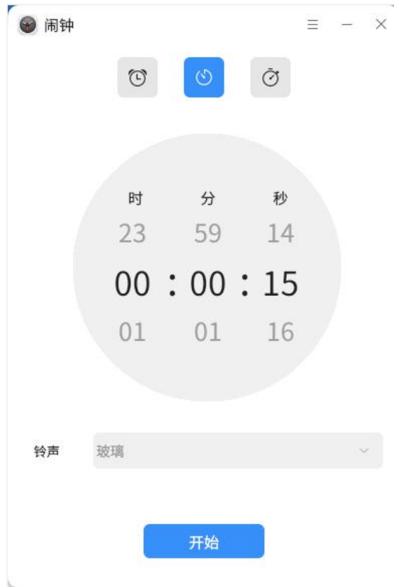
图 3.92 设定倒计时
