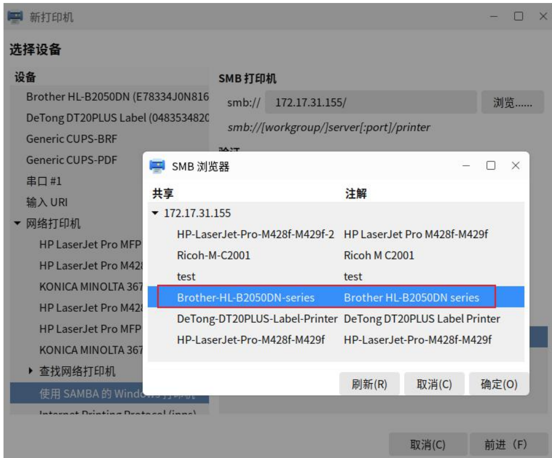
图 2.64 选择设备
