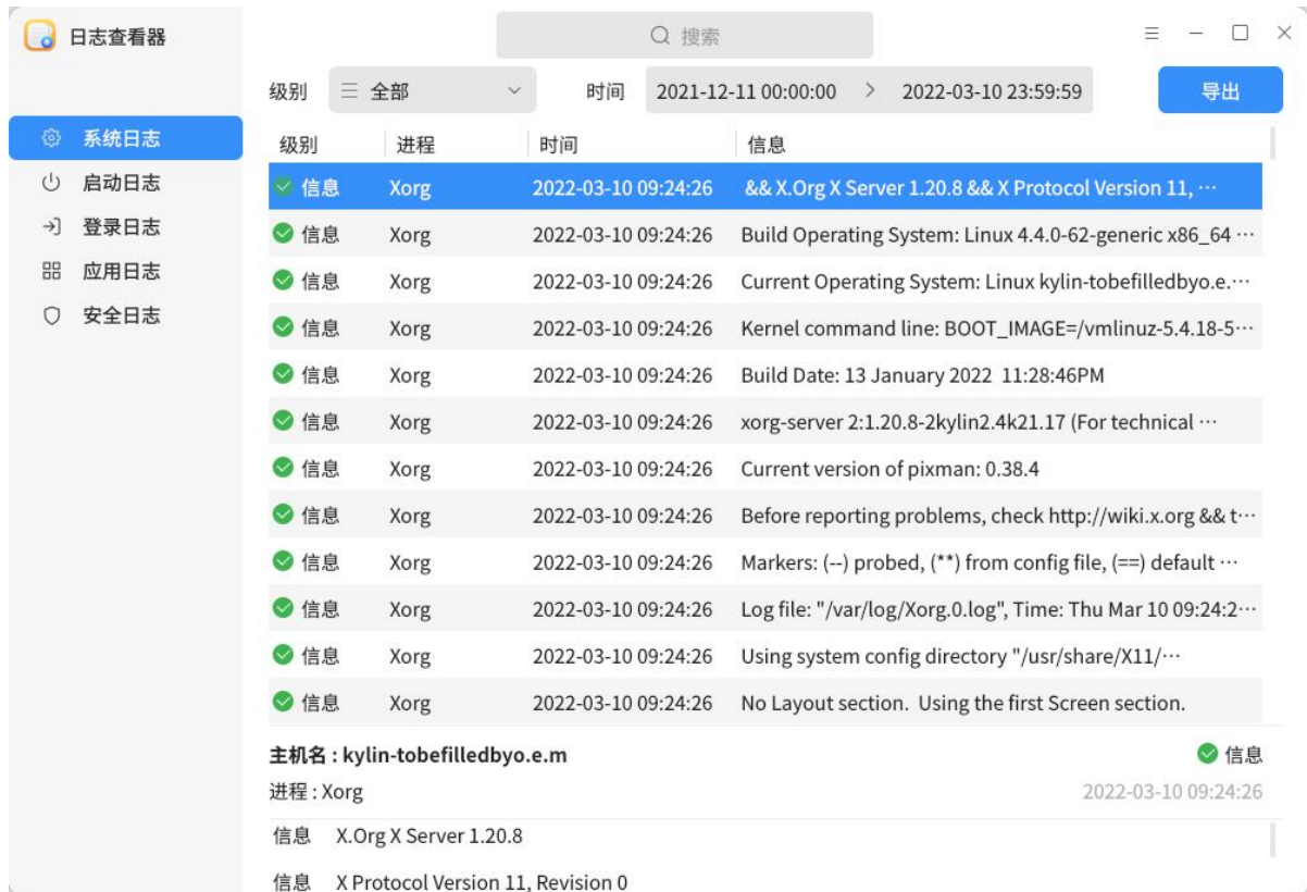
图 5.9 系统日志
