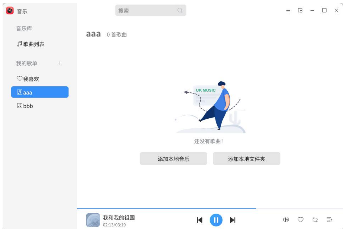
图 3.140 创建歌单
