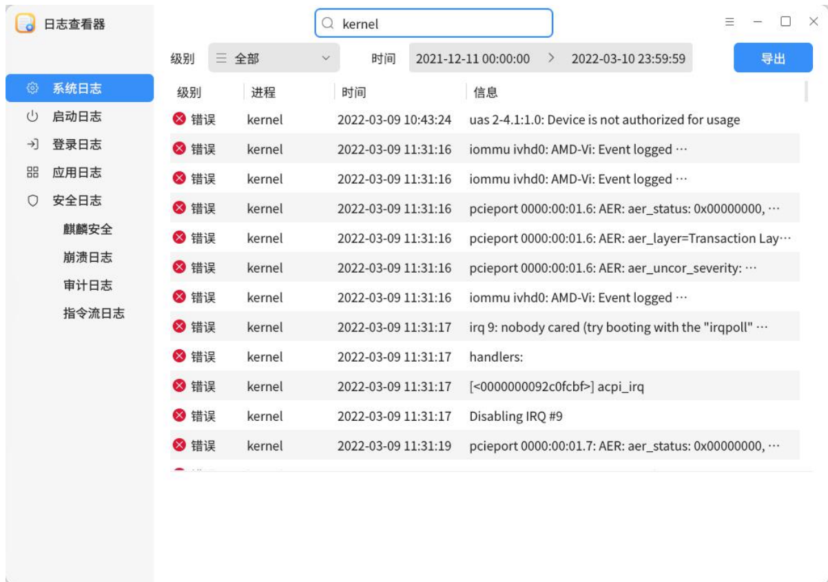
图 5.17 搜索操作
