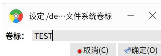
图 5.54 卷标
