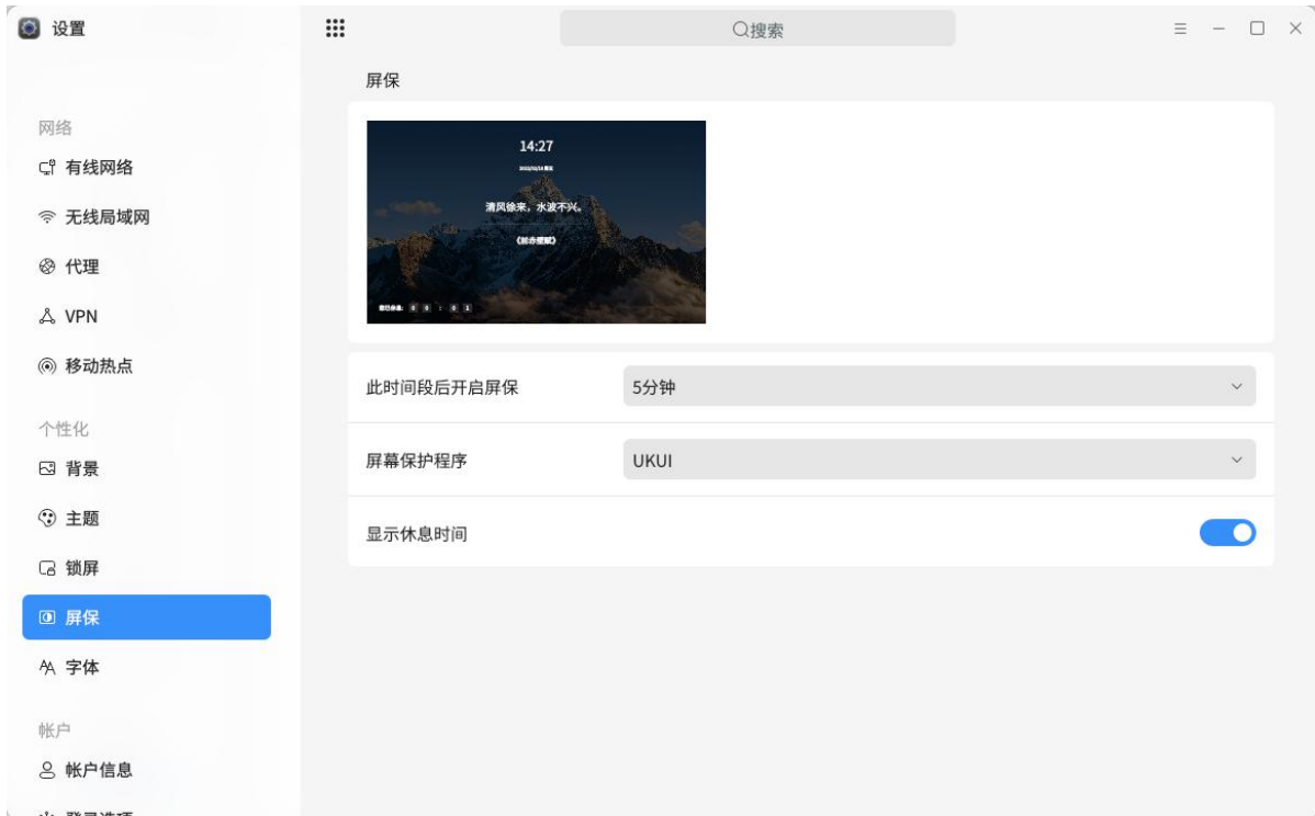
图 2.126 设置屏保
