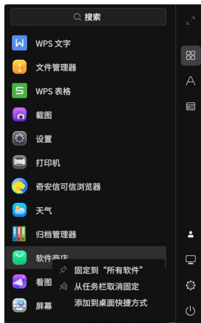
图 3.11 开始菜单
