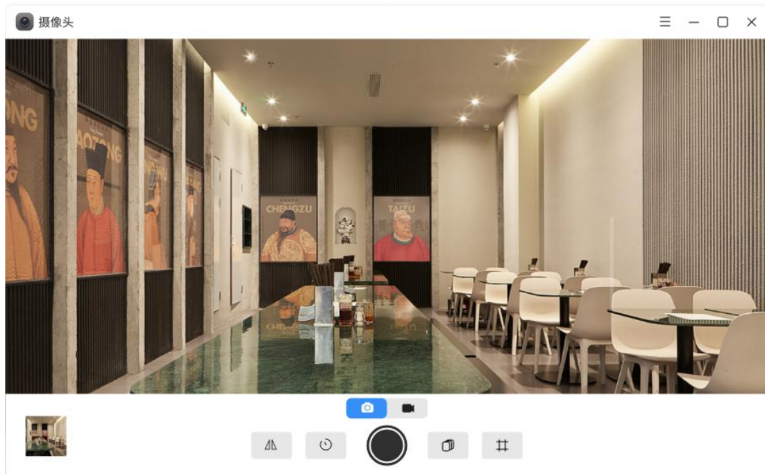
图 3.79 照相模式
