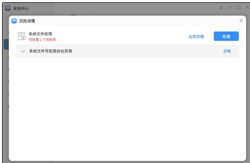
图 4.17 风险详情
