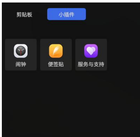
图 1.11 小插件
