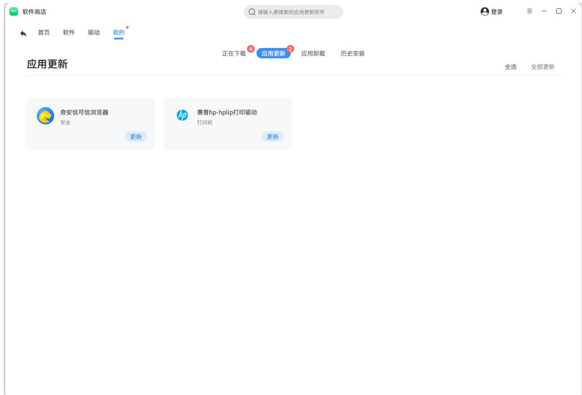
图 3.20 应用更新
