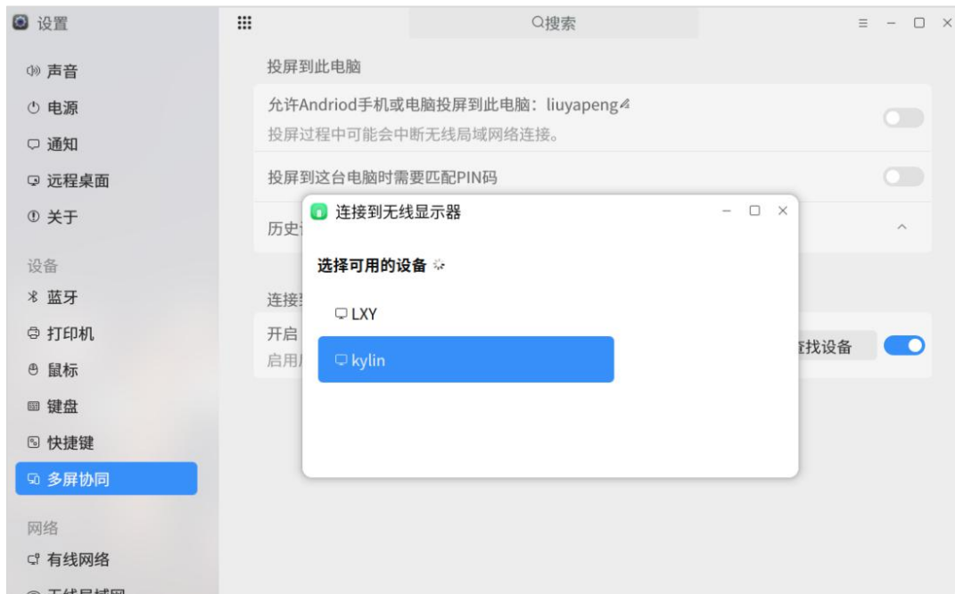
图 2.77 查找设备
