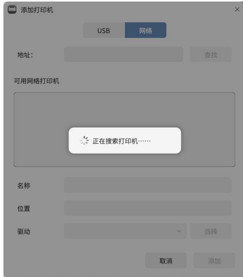
图 3.57 添加打印机
