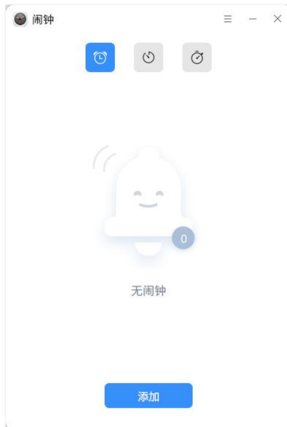
图 3.86 闹钟
