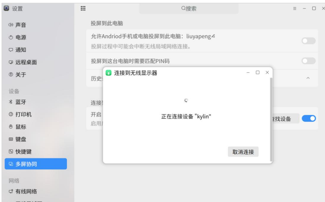
图 2.78 正在连接
