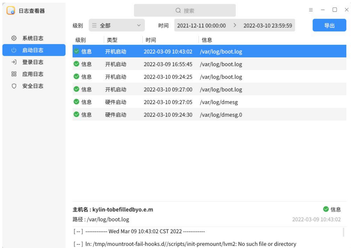
图 5.10 启动日志
