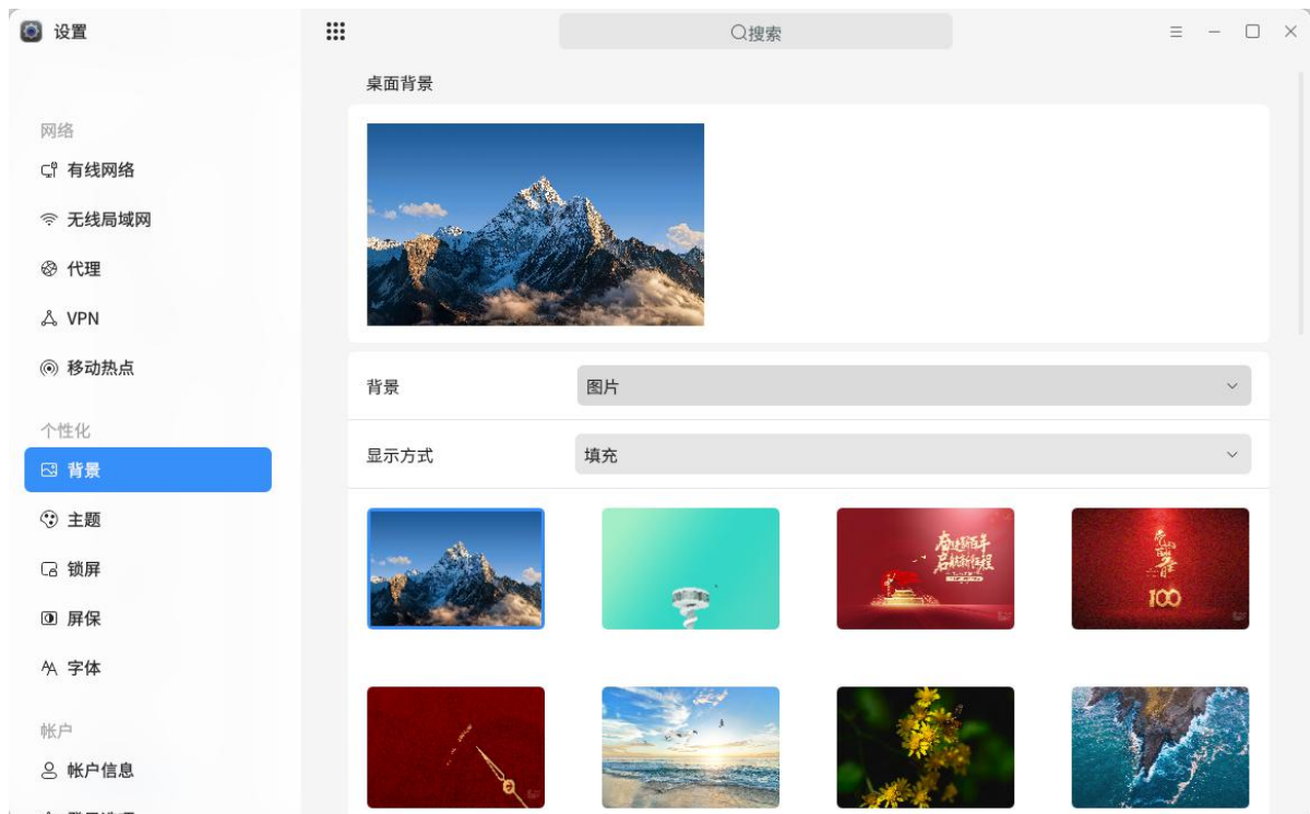
图 2.123 设置背景
