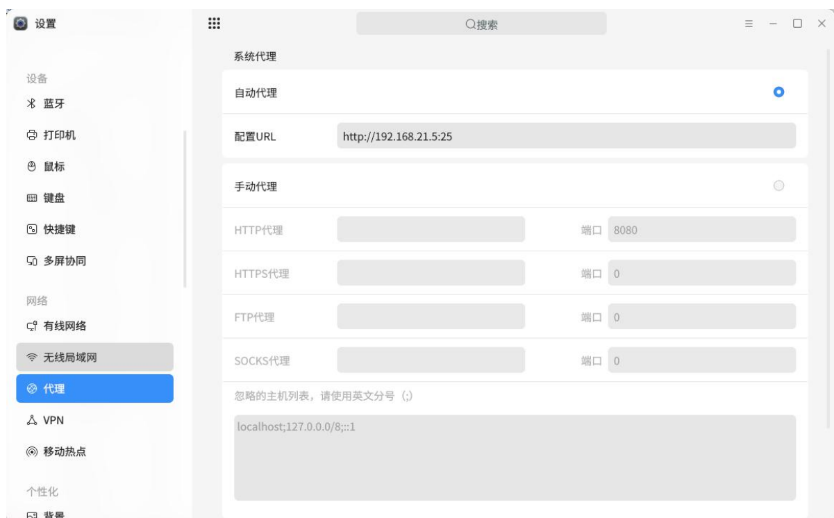
图 2.118 自动代理
